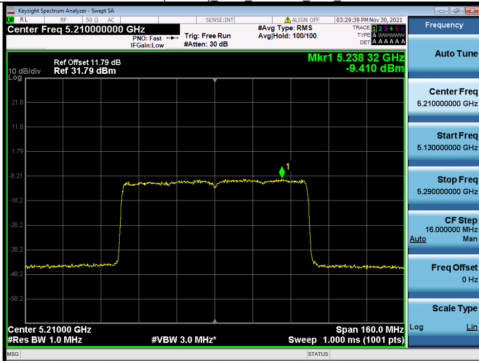
802.11ax(HEW80) MCH 5210MHz Ant2 NTN
