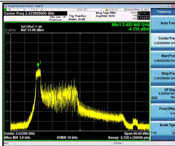
11AX40SISO_Ant2_2422_26Tone_RU8
