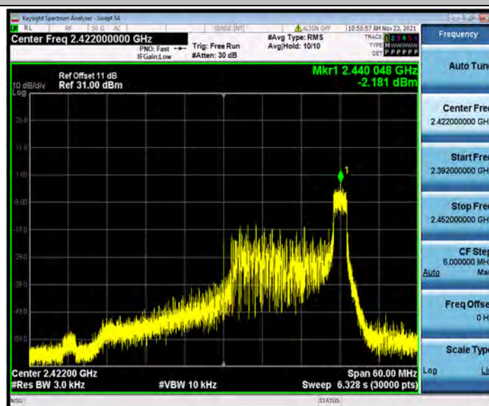
11AX40SISO_Ant1_2422_484Tone_RU65
