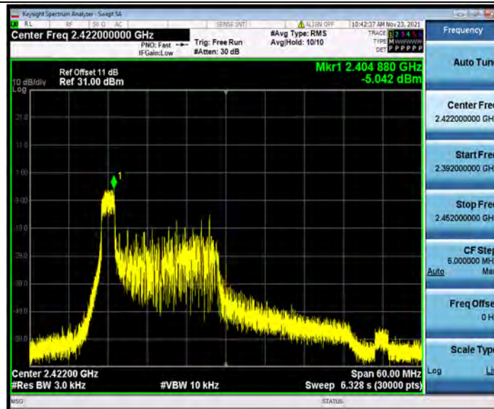
11AX40SISO_Ant1_2422_26Tone_RU8
