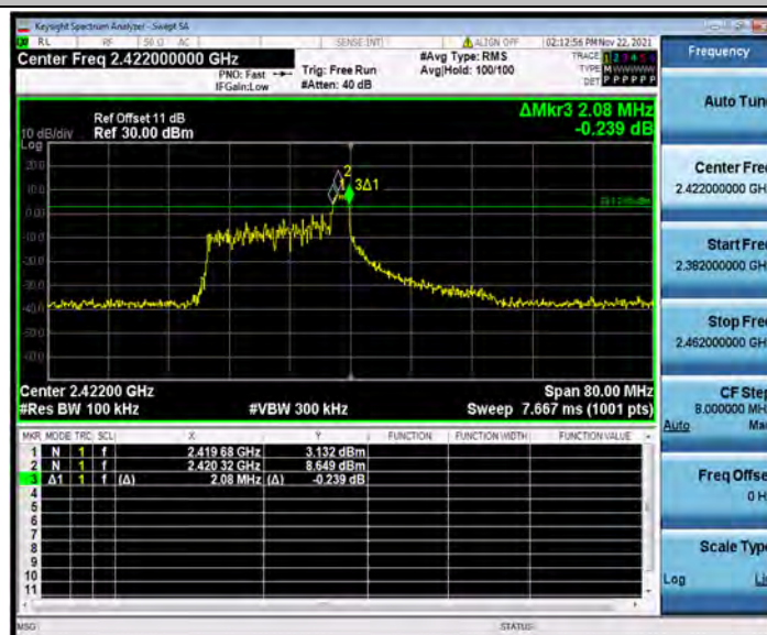
11AX40SISO_Ant2_2422_26Tone_RU17
