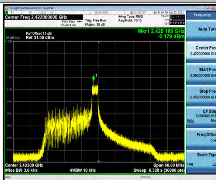
11AX40SISO_Ant1_2422_26Tone_RU17
