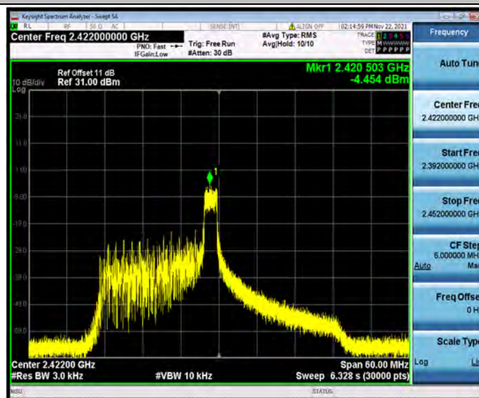
11AX40SISO_Ant2_2422_26Tone_RU17
