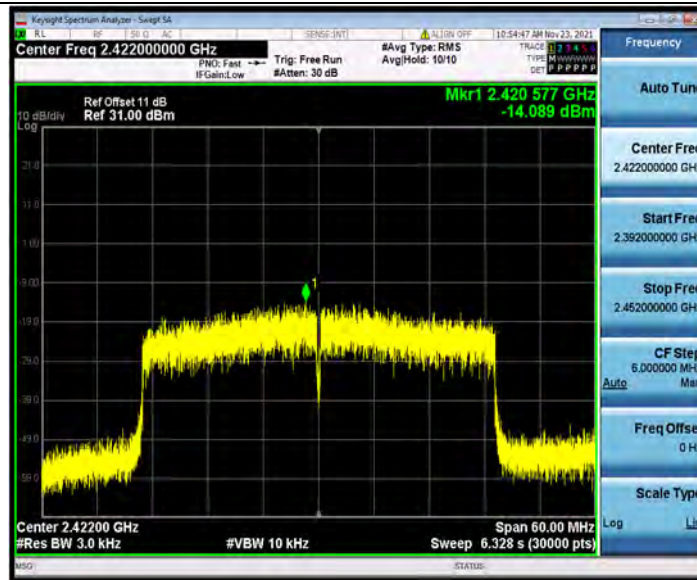
11AX40SISO_Ant2_2422_26Tone_RU0
