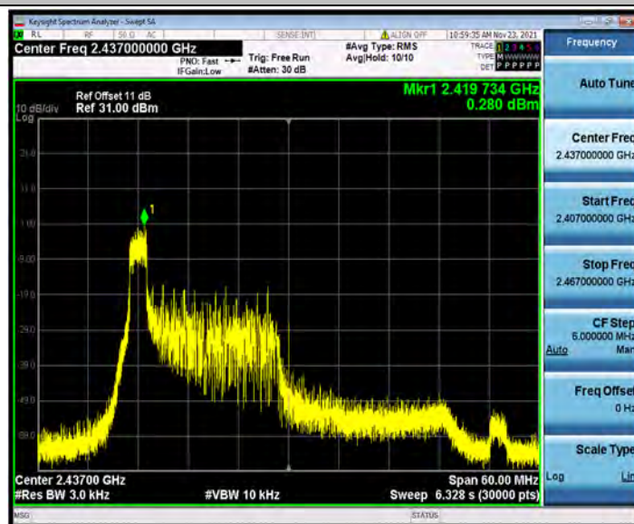
11AX40SISO_Ant1_2437_26Tone_RU8
