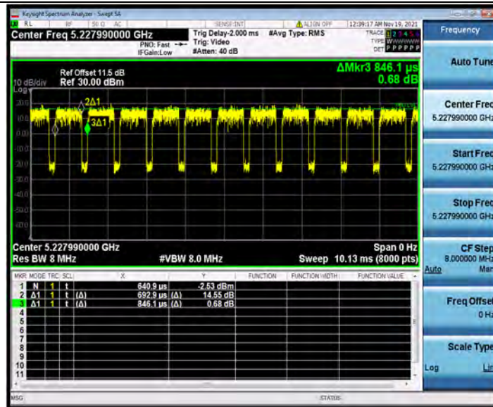
11AX40ISO_Ant2_5230_26Tone_RU17
