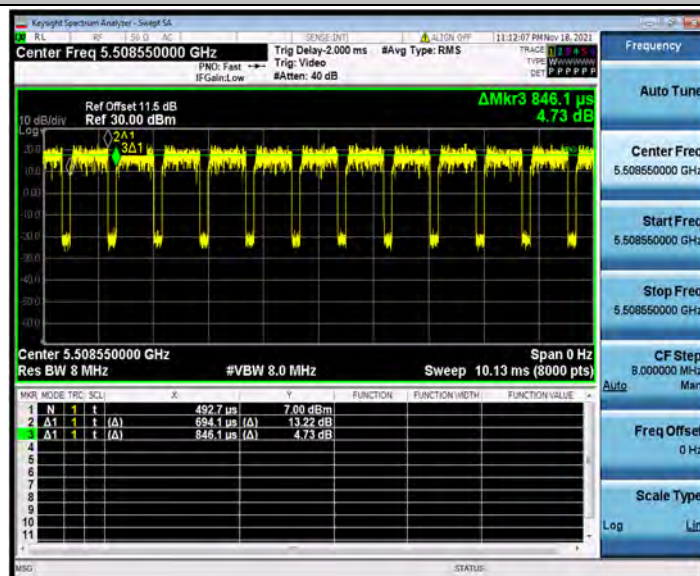
11AX20SISO_Ant2_5500_26Tone_RU5
