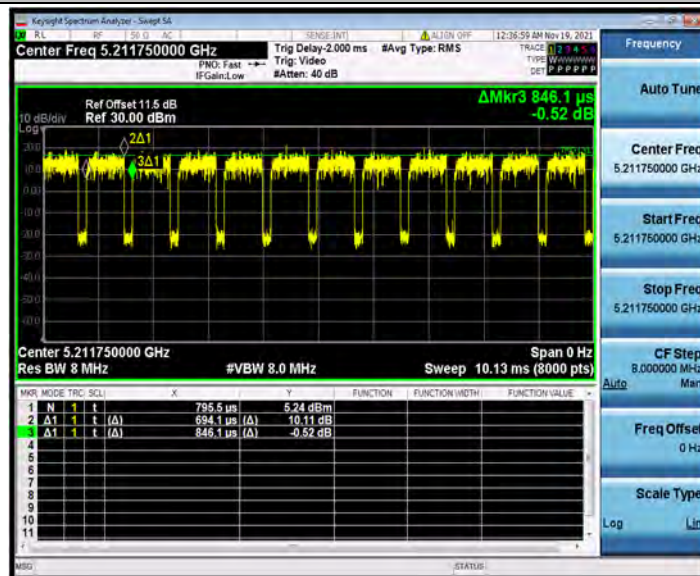
11AX40SISO_Ant2_5230_26Tone_RU8
