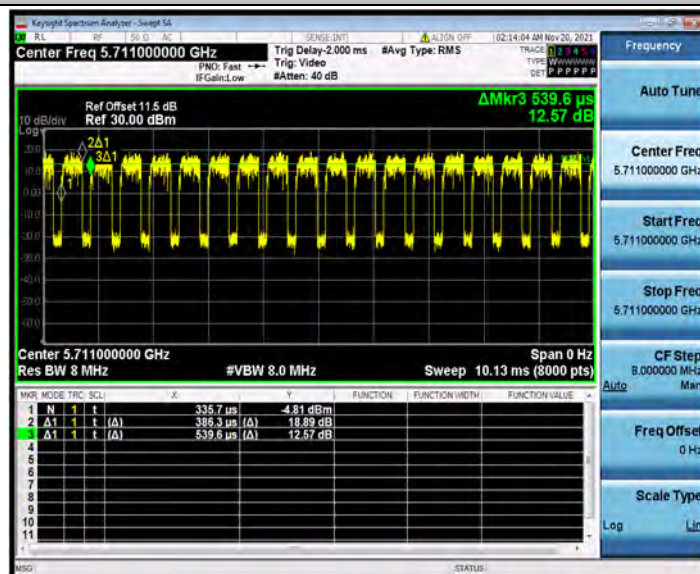
11AX20MIMO_Ant1_5720_26Tone_RU0
