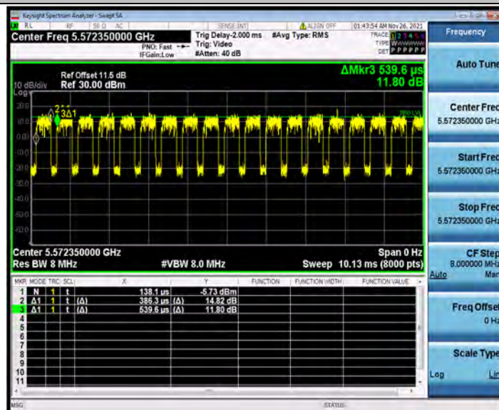
11AX20MIMO_Ant1_5580_26Tone_RU4
