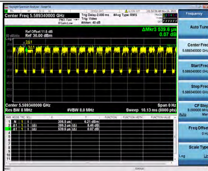
11AX20MIMO_Ant2_5580_26Tone_RU8
