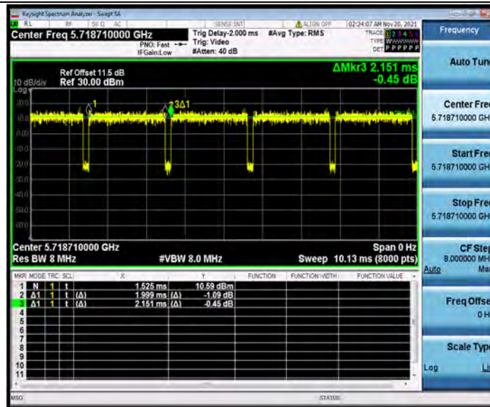
11AX20MIMO_Ant2_5720_26Tone_RU0
