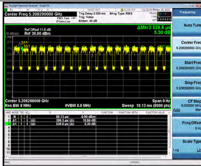
11AX20MIMO_Ant1_5200_242Tone_RU61
