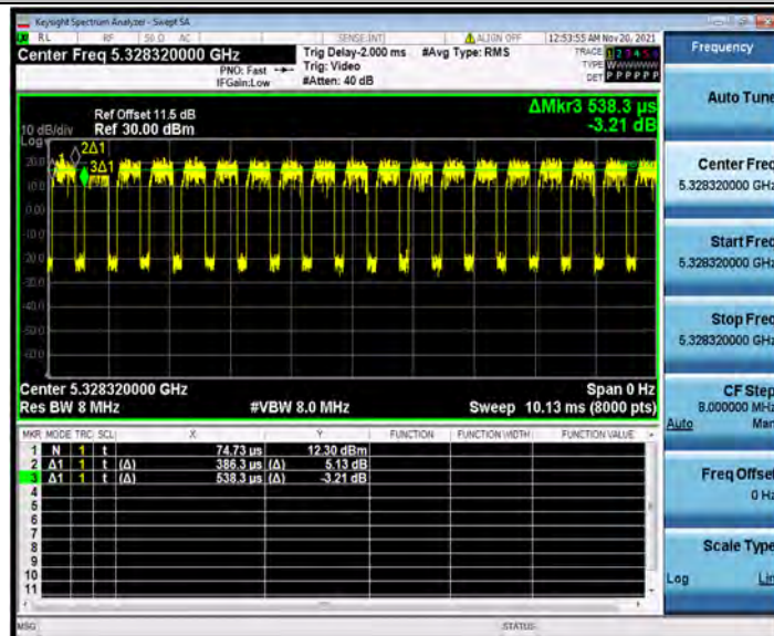
11AX20MIMO_Ant2_5320_242Tone_RU61
