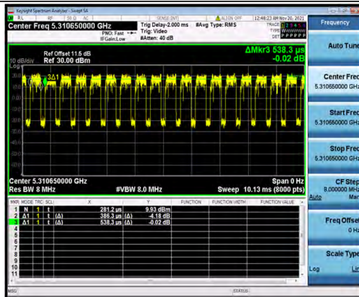
11AX20MIMO_Ant2_5320_26Tone_RU4
