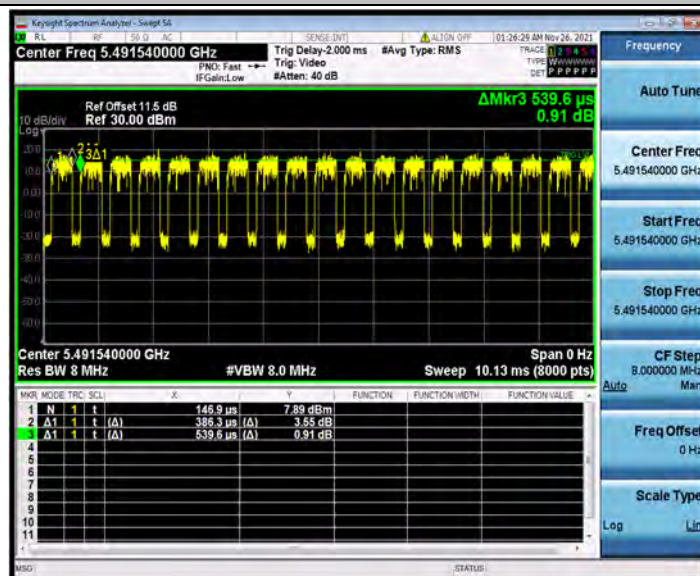
11AX20MIMO_Ant2_5500_26Tone_RU0
