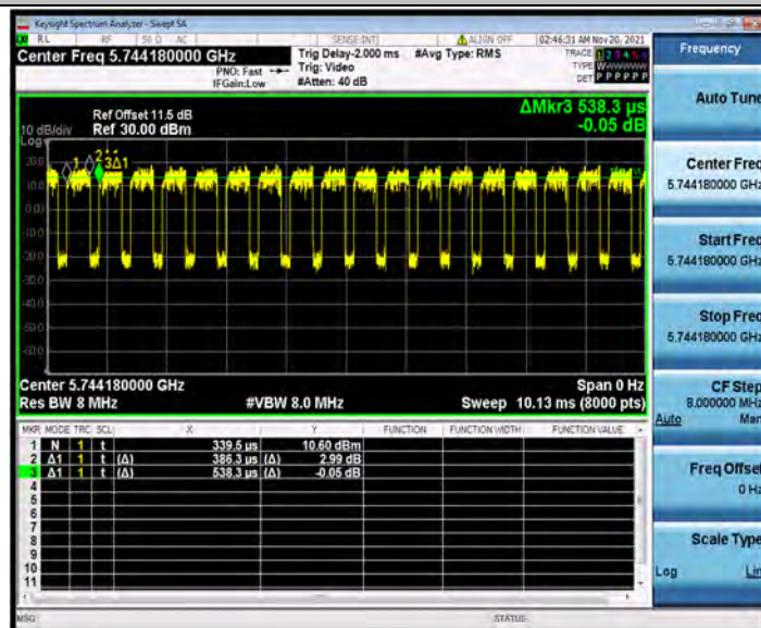
11AX20MIMO_Ant1_5745_26Tone_RU8
