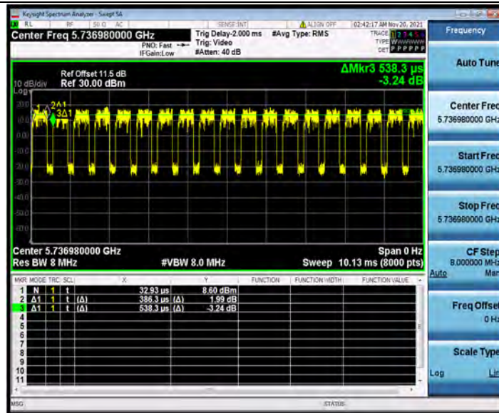
11AX20MIMO_Ant1_5745_26Tone_RU4
