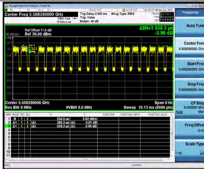
11AX20MIMO_Ant1_5500_242Tone_RU61
