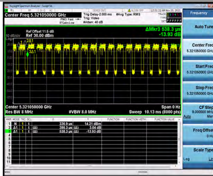
11AX20MIMO_Ant2_5320_26Tone_RU8
