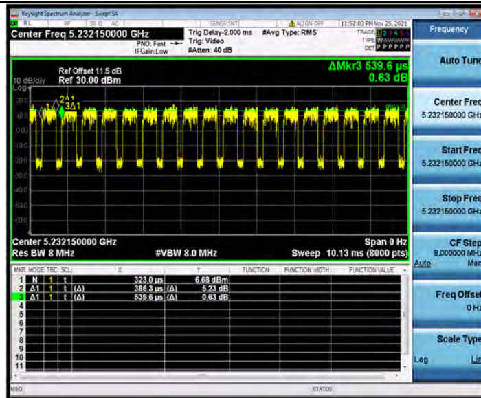
11AX20MIMO_Ant2_5240_26Tone_RU4
