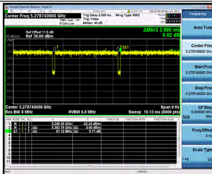
11AX80SISO_Ant2_5290_996Tone_RU67
