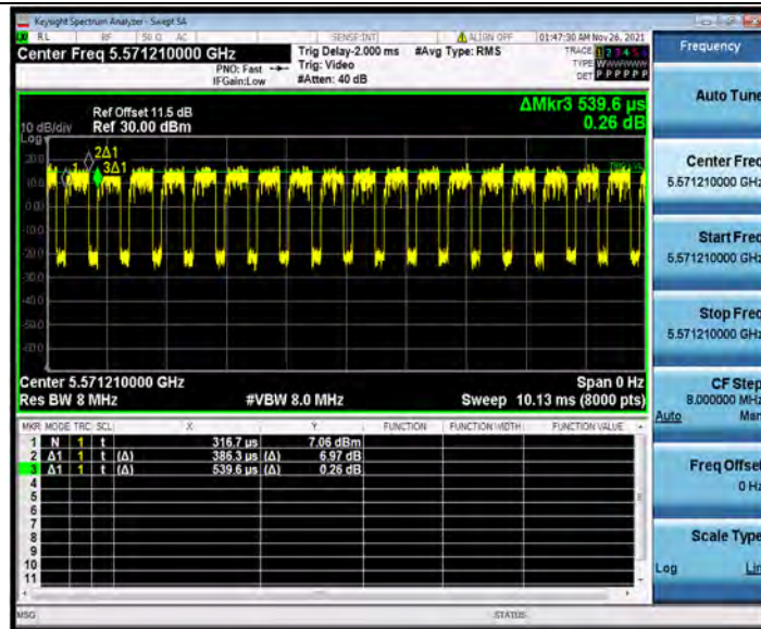
11AX20MIMO_Ant2_5580_26Tone_RU4
