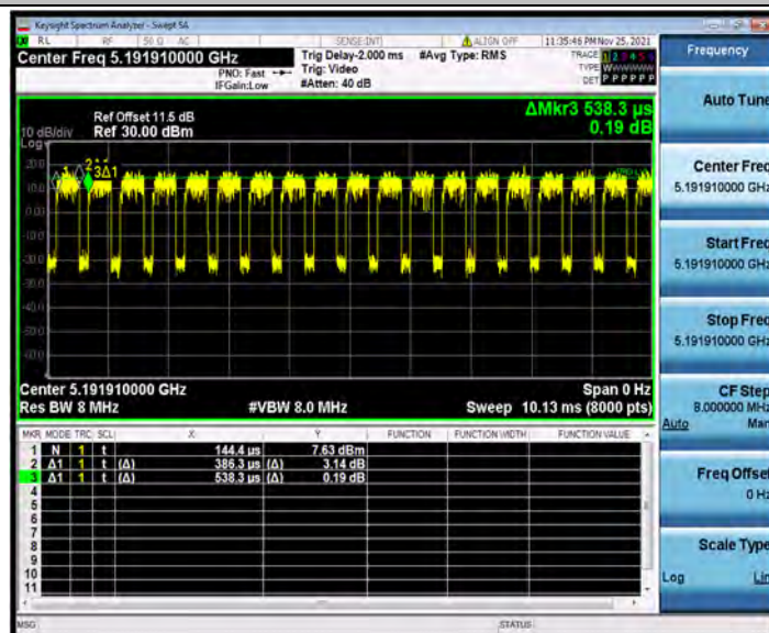
11AX20MIMO_Ant2_5200_26Tone_RU0
