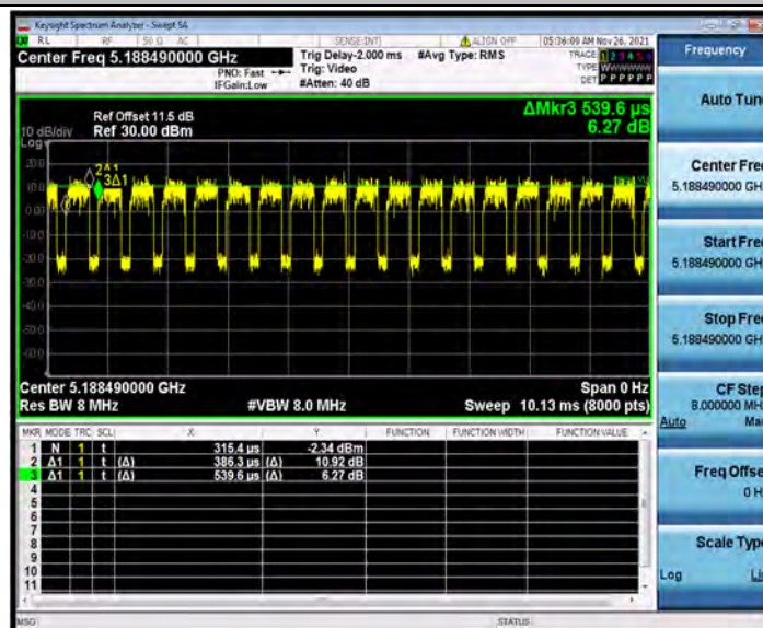
11AX20MIMO_Ant1_5180_26Tone_RU8
