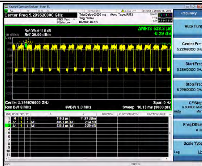
11AX20MIMO_Ant2_5300_26Tone_RU4
