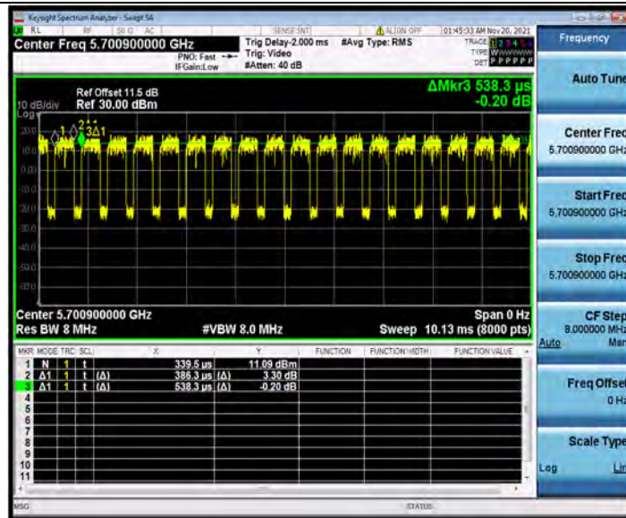
11AX20MIMO_Ant1_5700_26Tone_RU8
