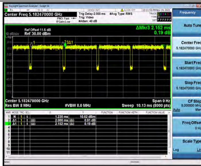
11AX20MIMO_Ant2_5180_26Tone_RU0
