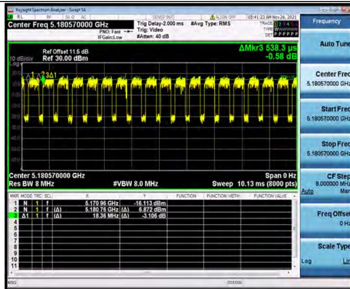
11AX20MIMO_Ant2_5180_26Tone_RU8
