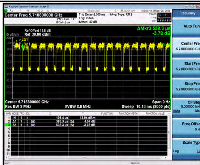
11AX20MIMO_Ant2_5720_26Tone_RU4
