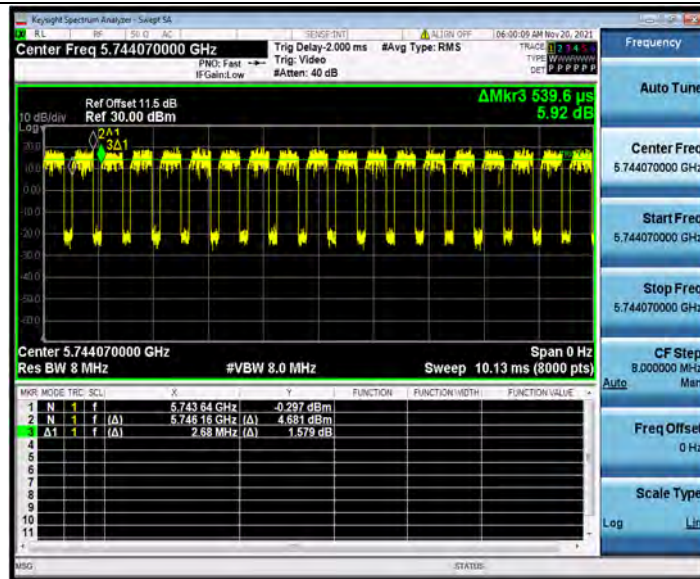
11AX20MIMO_Ant2_5745_26Tone_RU8
