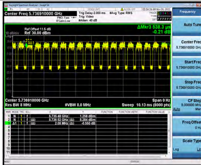
11AX20MIMO_Ant2_5745_26Tone_RU4
