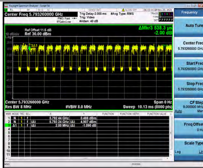
11AX20MIMO_Ant1_5785_242Tone_RU61
