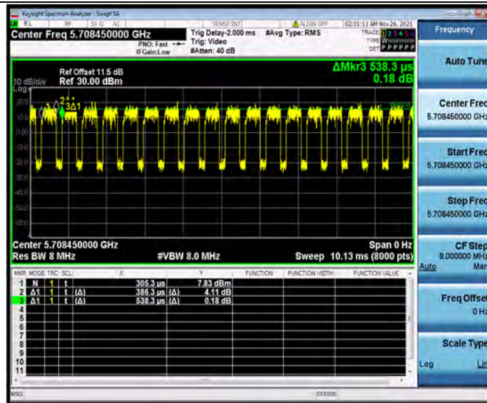
11AX20MIMO_Ant2_5700_242Tone_RU61
