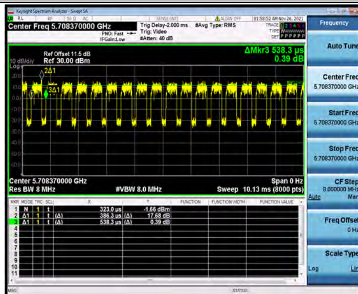
11AX20MIMO_Ant1_5700_242Tone_RU61
