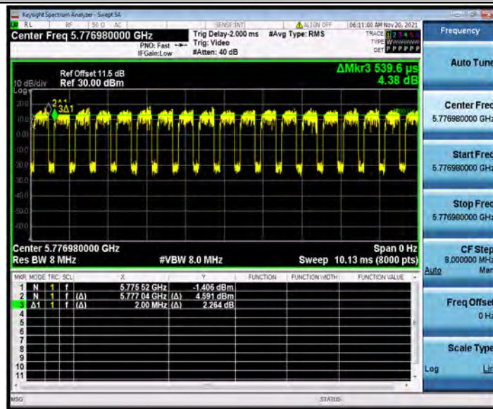
11AX20MIMO_Ant1_5785_26Tone_RU4
