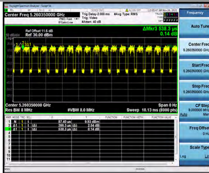
11AX20MIMO_Ant1_5260_26Tone_RU8
