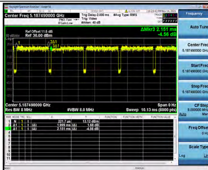
11AX20MIMO_Ant2_5180_242Tone_RU61
