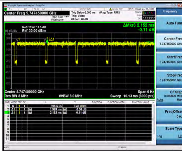
11AX20MIMO_Ant2_5745_26Tone_RU0
