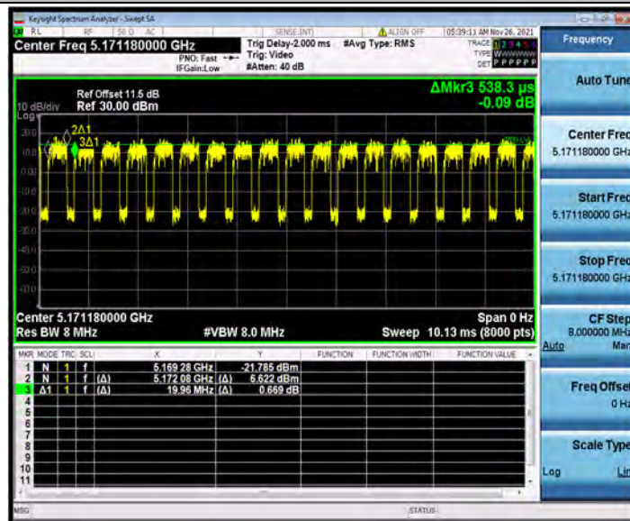
11AX20MIMO_Ant2_5180_26Tone_RU4
