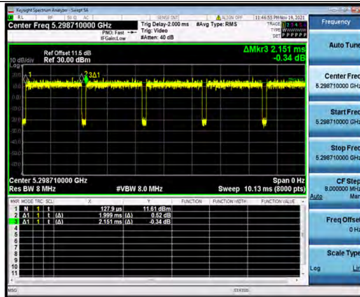
11AX20MIMO_Ant2_5300_26Tone_RU0
