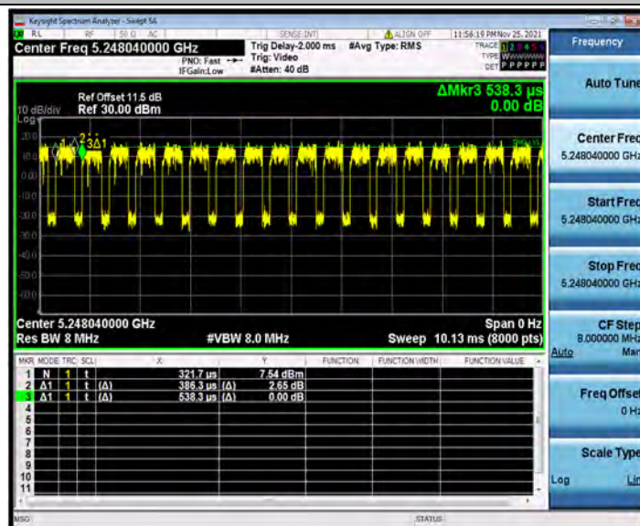
11AX20MIMO_Ant2_5240_26Tone_RU8
