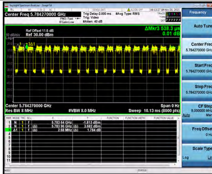
11AX20MIMO_Ant1_5785_26Tone_RU8
