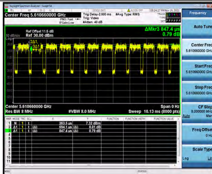
11AX80ISO_Ant2_5610_26Tone_RU36
