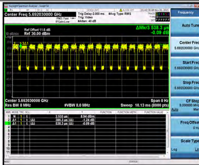
11AX20MIMO_Ant1_5700_26Tone_RU4
