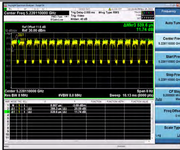
11AX40MIMO_Ant1_5230_26Tone_RU17
