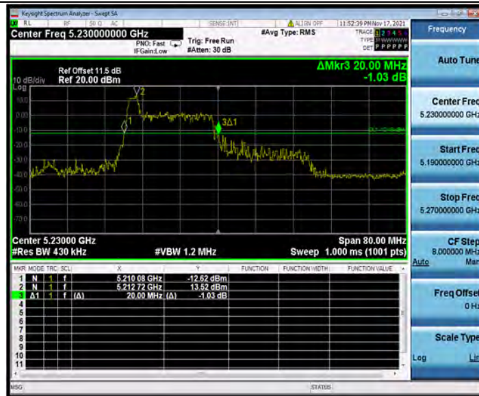
11AX40SISO_Ant1_5230_26Tone_RU8
