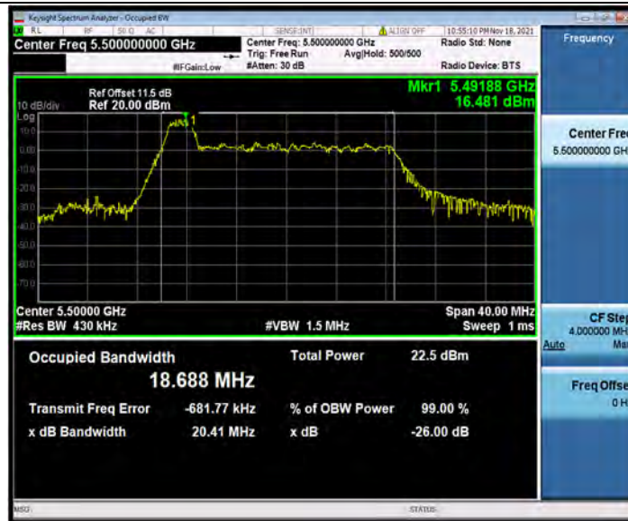
11AX20SISO_Ant2_5500_26Tone_RU4
