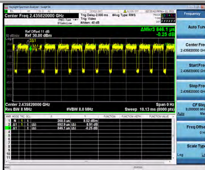
11AX40SISO_Ant2_2437_26Tone_RU17
