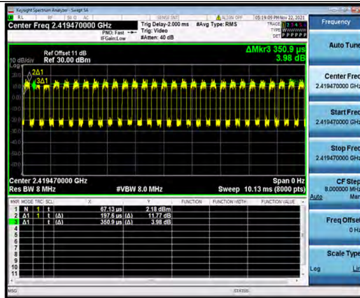
11AX40MIMO_Ant2_2422_26Tone_RU0
