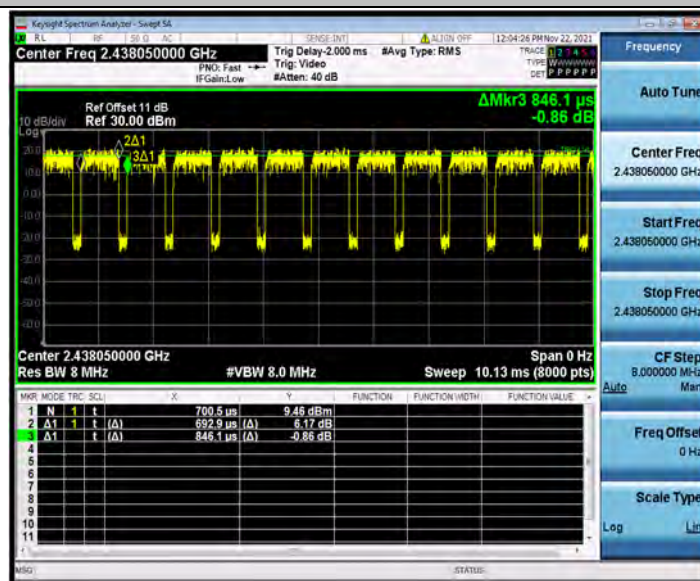
11AX20SISO_Ant2_2437_26Tone_RU6
