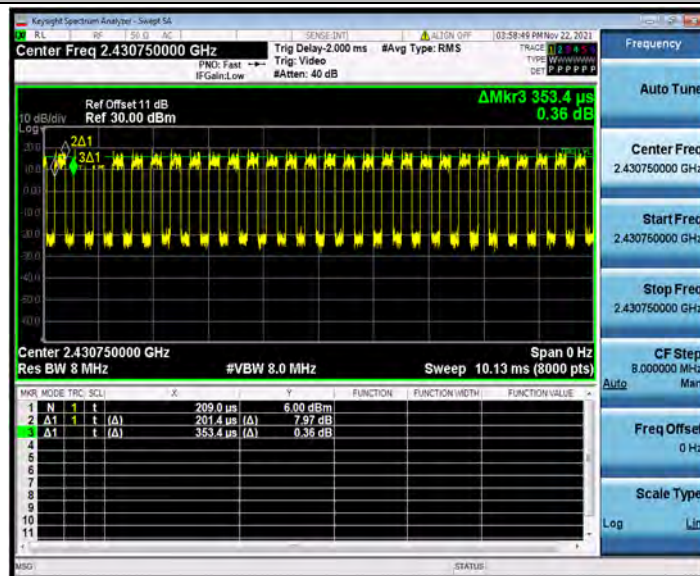
11AX20MIMO_Ant2_2437_26Tone_RU0
