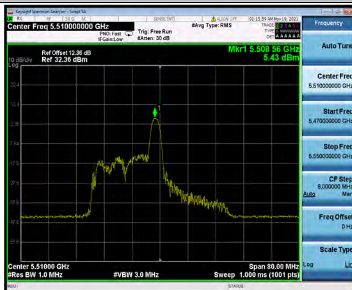
11AX40SISO_Ant2_5510_26Tone_RU0
