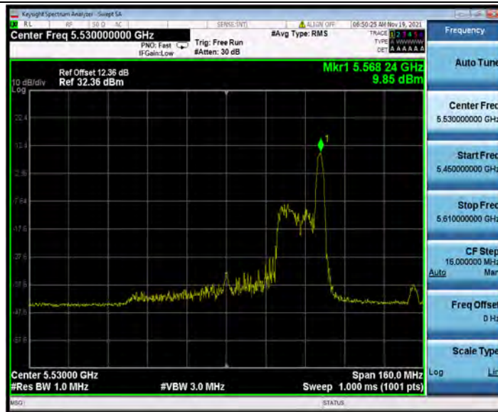
11AX80SISO_Ant2_5530_996Tone_RU67
