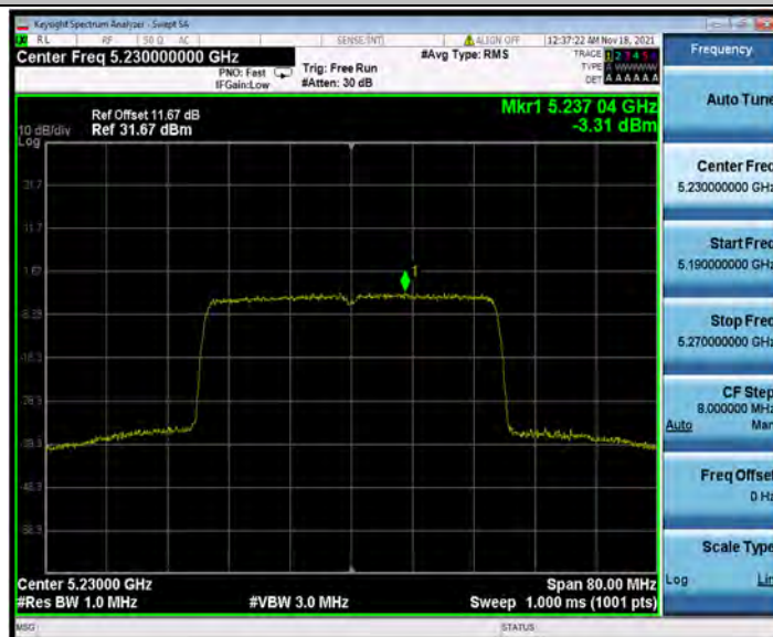
11AX40SISO_Ant2_5230_26Tone_RU0
