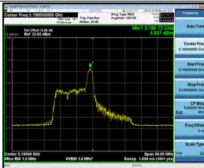
11AX40MIMO_Ant2_5190_26Tone_RU17
