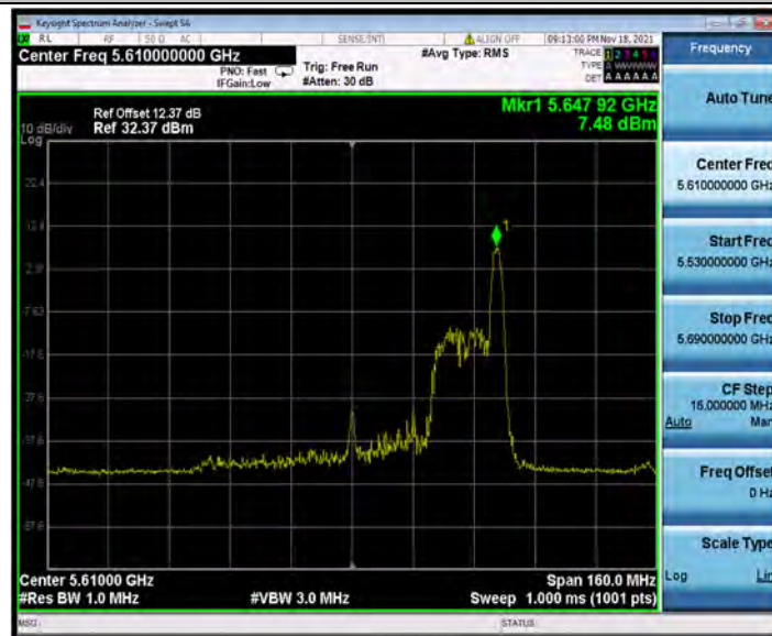
11AX80SISO_Ant1_5610_996Tone_RU67
