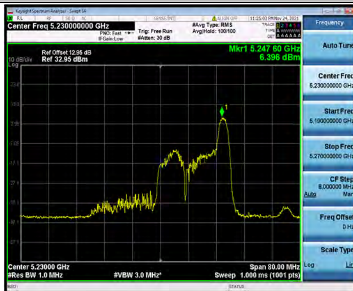
11AX40MIMO_Ant1_5230_484Tone_RU65
