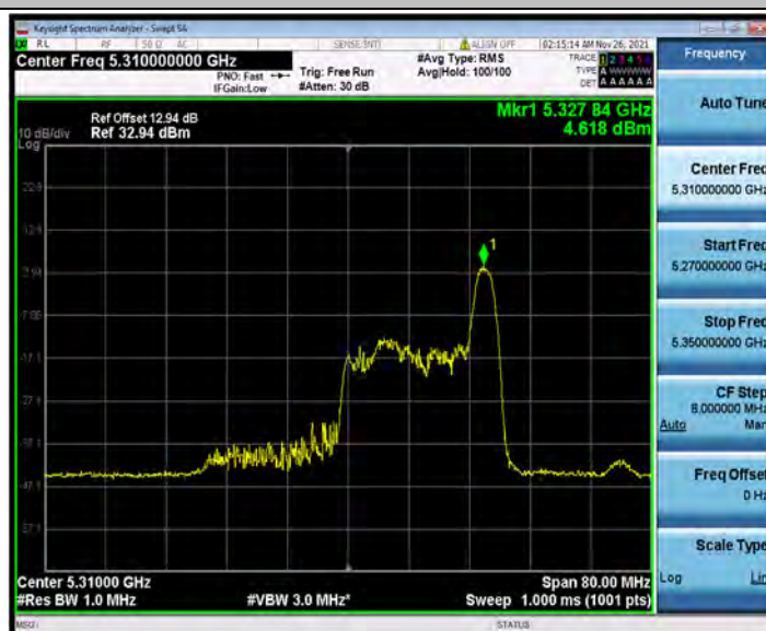
11AX40MIMO_Ant1_5310_26Tone_RU17
