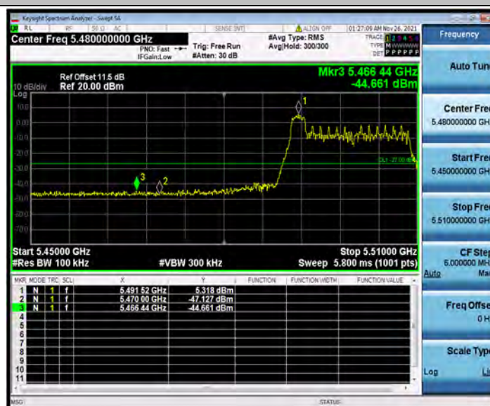
11AX20MIMO_Ant2_Low_5500_26Tone_RU0
