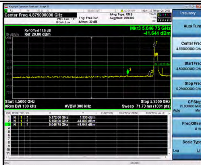
11AX80MIMO_Ant2_Low_5210_26Tone_RU0
