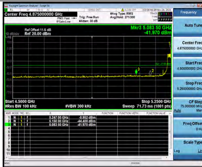
11AX80MIMO_Ant1_Low_5210_996Tone_RU67
