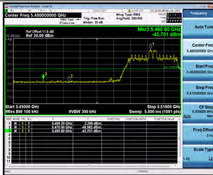
11AX20MIMO_Ant1_Low_5500_26Tone_RU8
