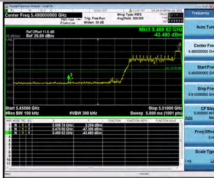
11AX20MIMO_Ant1_Low_5500_242Tone_RU61
