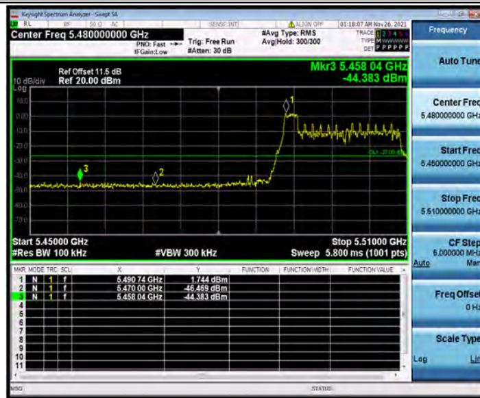
11AX20MIMO_Ant1_Low_5500_26Tone_RU4
