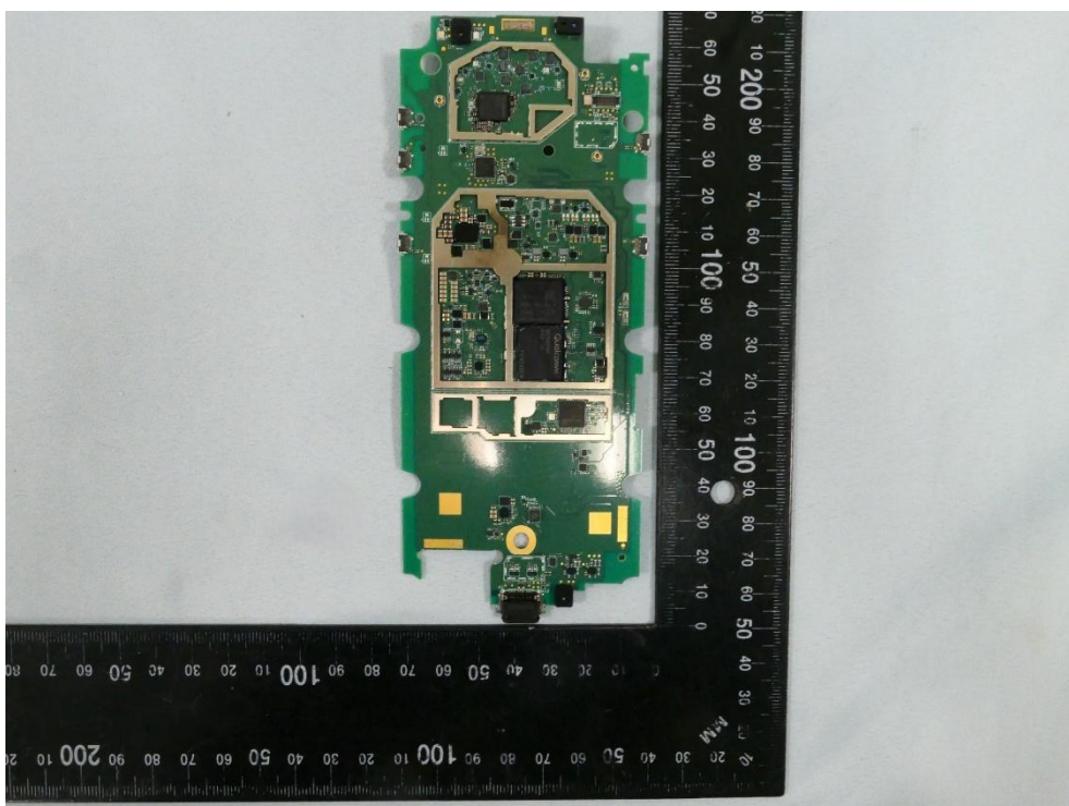
(10) EUT Photo (S0703)
