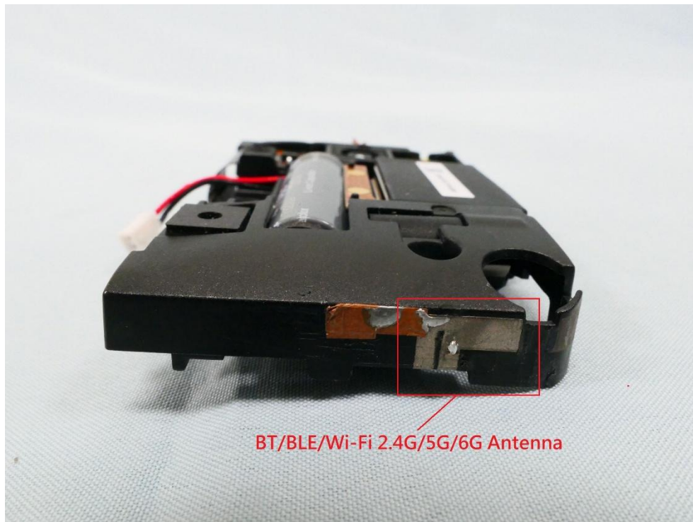
(24) EUT Photo (S0803FR)
