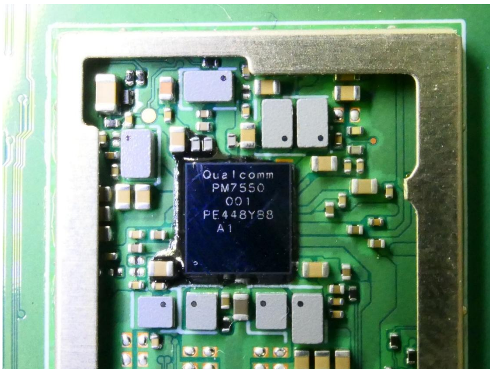
(32) EUT Photo (S0803FR)
