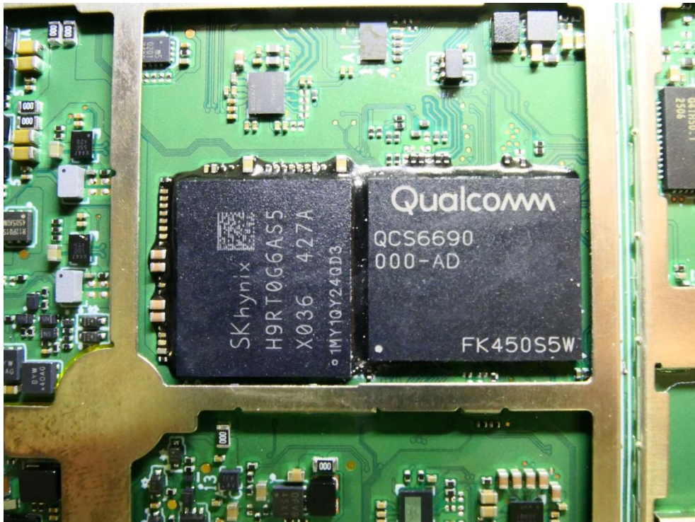
(12) EUT Photo (S0703)
