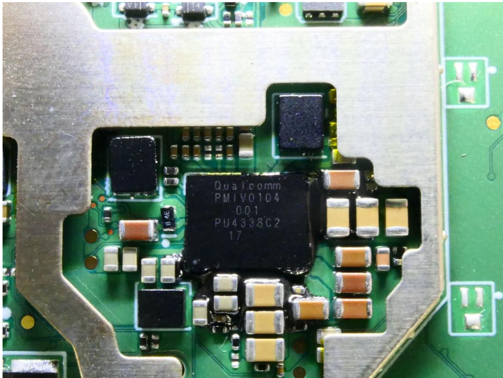
(30) EUT Photo (S0803FR)
