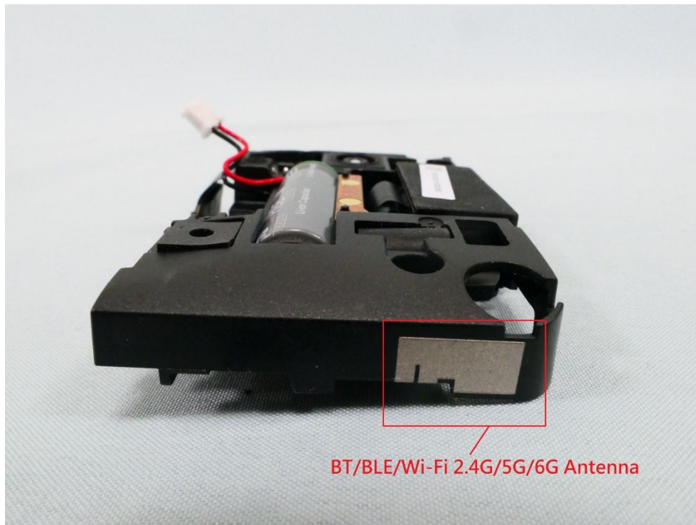
(8) EUT Photo (S0703)
