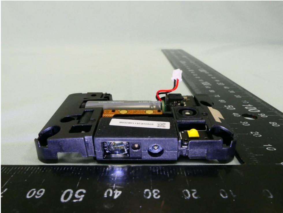
(6) EUT Photo (S0703)
