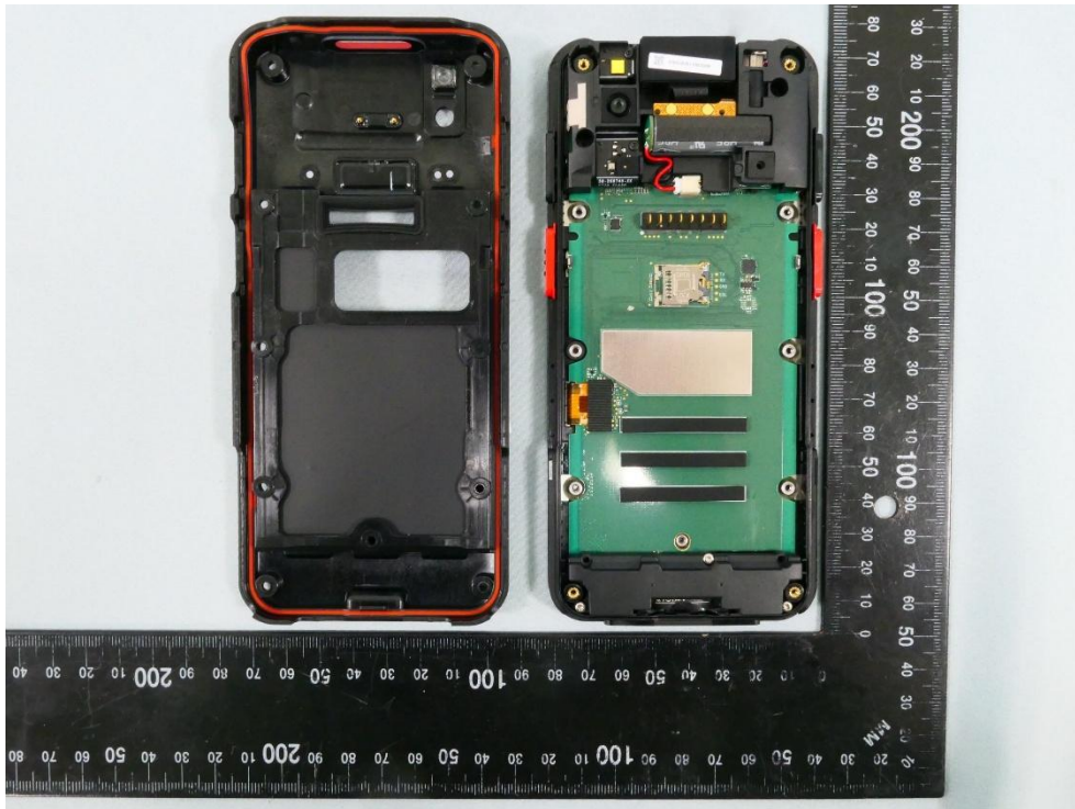
(2) EUT Photo (S0703)
