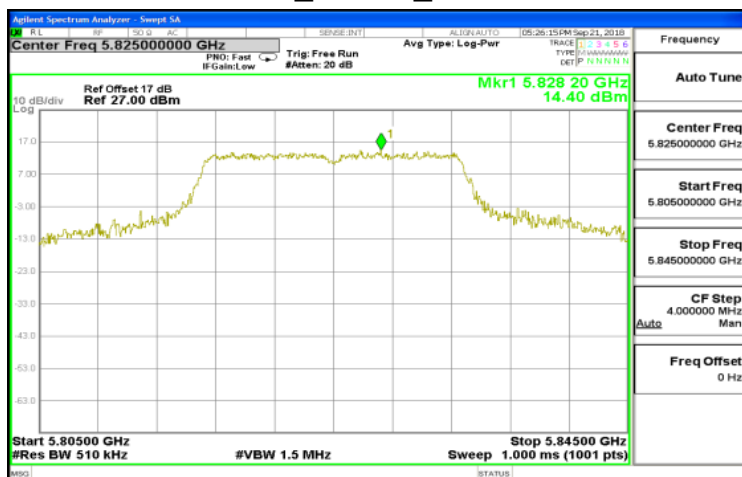
802.11n_20MHz_5825MHz
