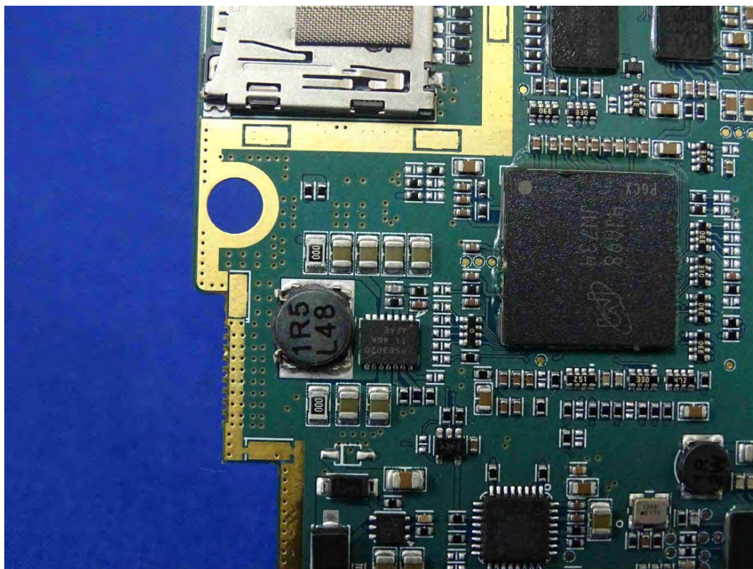
(33) EUT Photo
