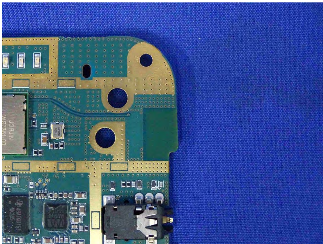
(37) EUT Photo
