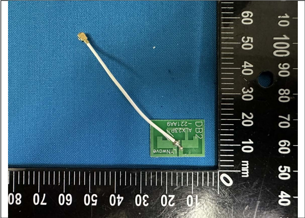
2.4G+5G ant 1
