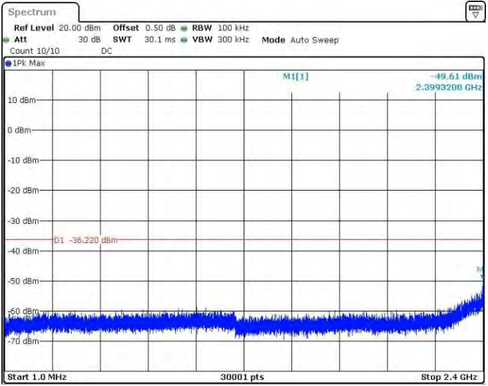
11N40SISO_Ant2_2422_1~2400
