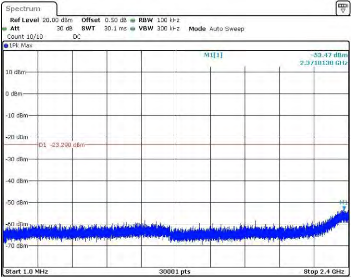
11B_Ant2_2462_1~2400
