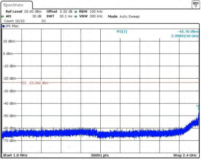
11B_Ant1_2412_1~2400
