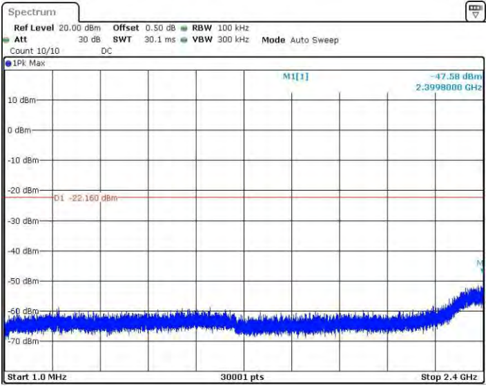
11GMINO_Ant3_2412_1~2400
