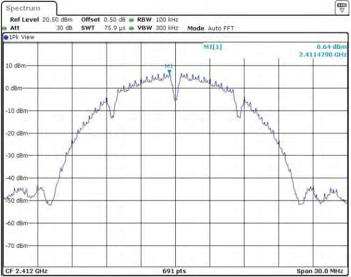
11B_Ant1_2412_0~Reference
