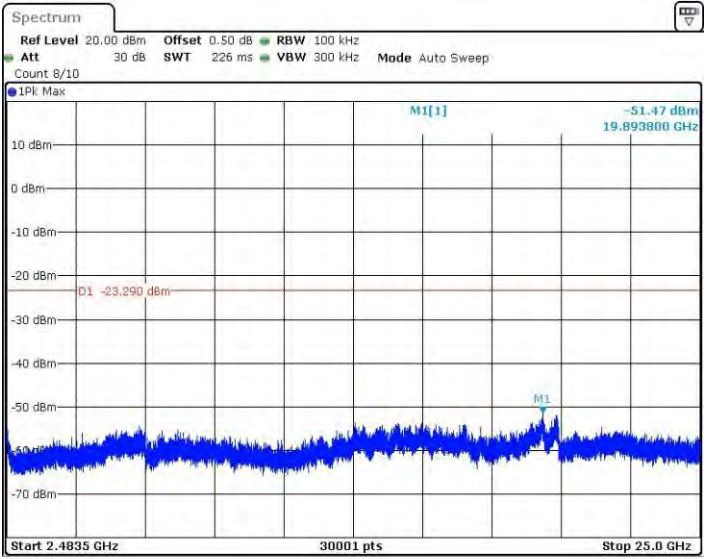
11B_Ant2_2462_2483.5~25000
