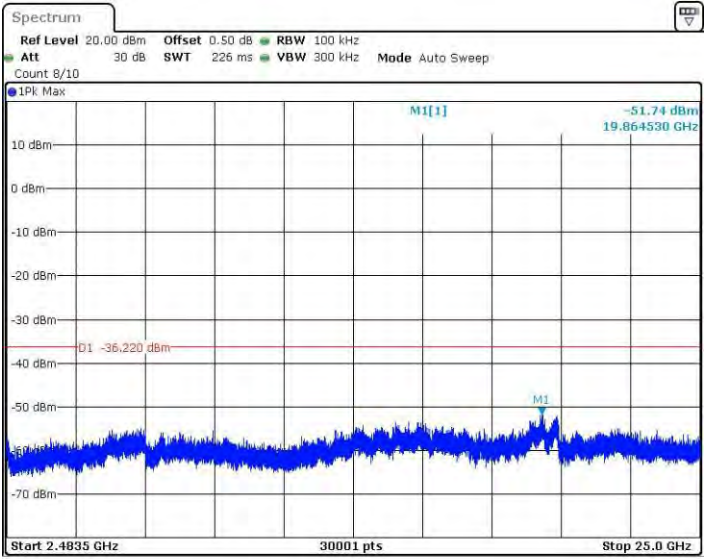
11N40SISO_Ant2_2422_2483.5~25000
