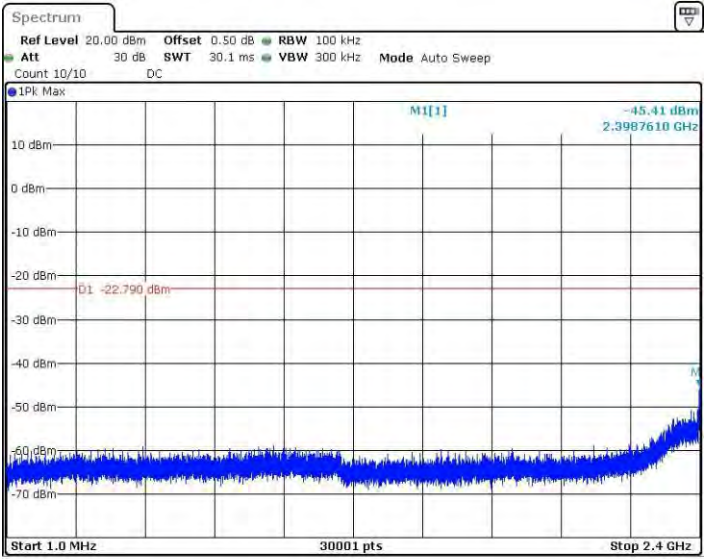
11B_Ant4_2412_1~2400
