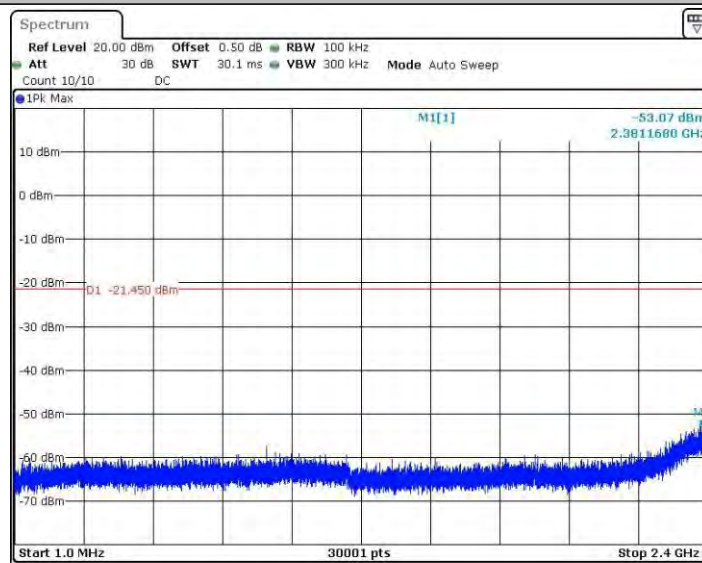
11GMINO_Ant2_2462_0-Reference
