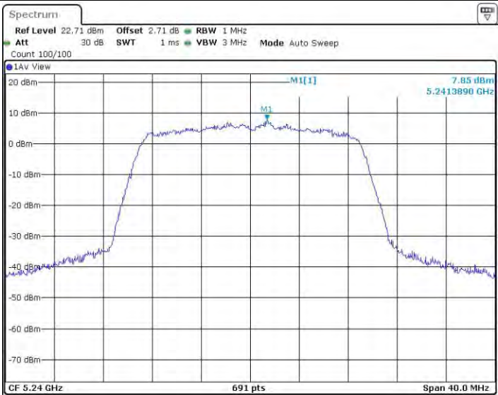
11N20BF_Ant1_5240
