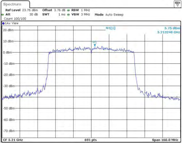
11AC80MIMO_Ant2_5210
