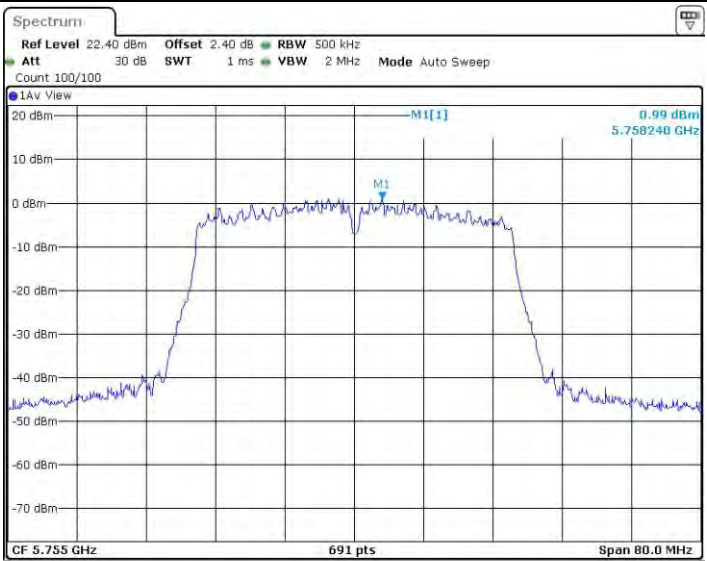
11N40BF_Ant2_5755
