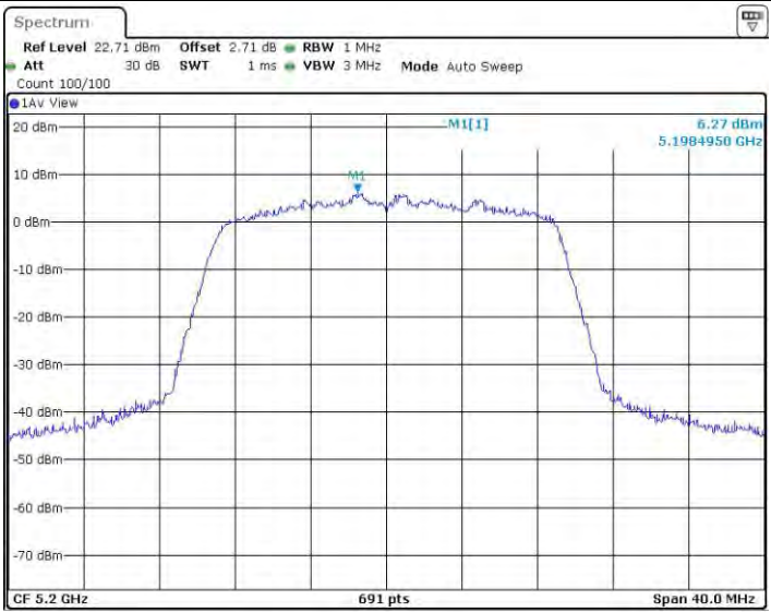
11N20BF_Ant2_5200
