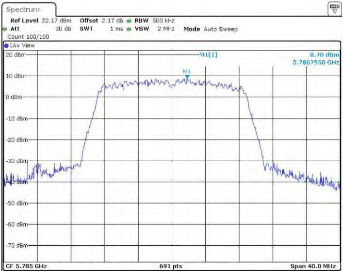
11N20MIMO_Ant3_5785
