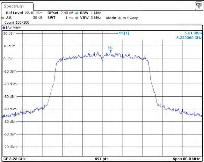
11N40BF_Ant3_5230
