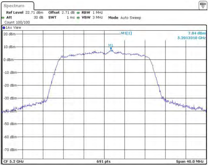
11N20BF_Ant1_5200
