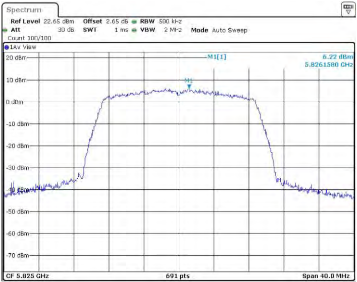
11AC20MIMO_Ant4_5825
