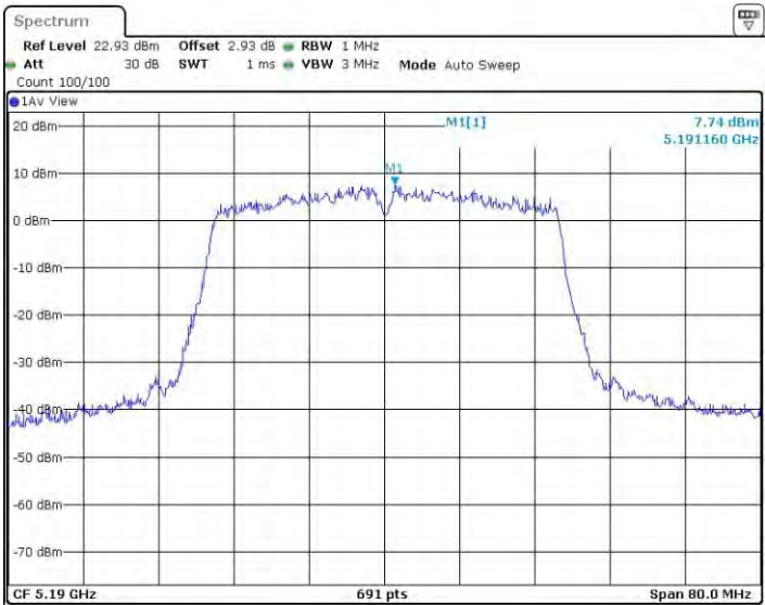
11AC40MIMO_Ant3_5190
