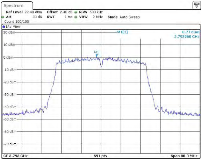
11N40BF_Ant1_5795
