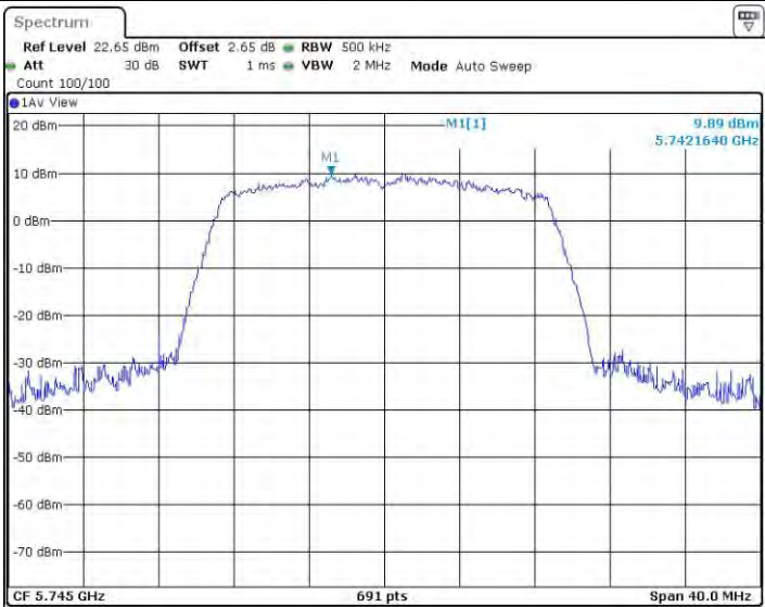
11AC20MIMO_Ant4_5745
