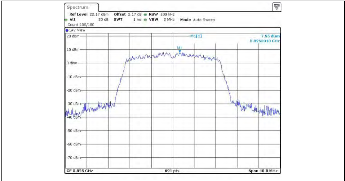
11N20MIMO_Ant1_5825
