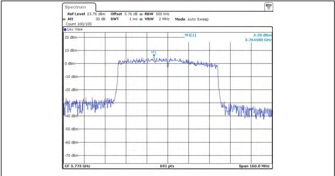
11AC80MIMO_Ant3_5775
