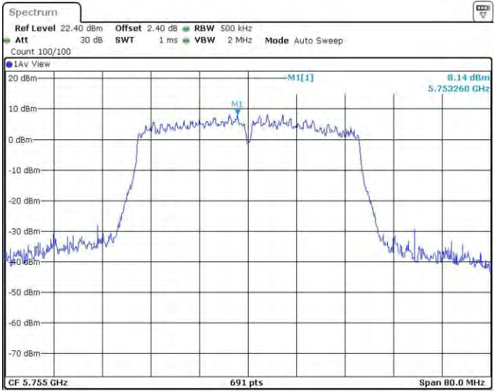
11N40MIMO_Ant3_5755
