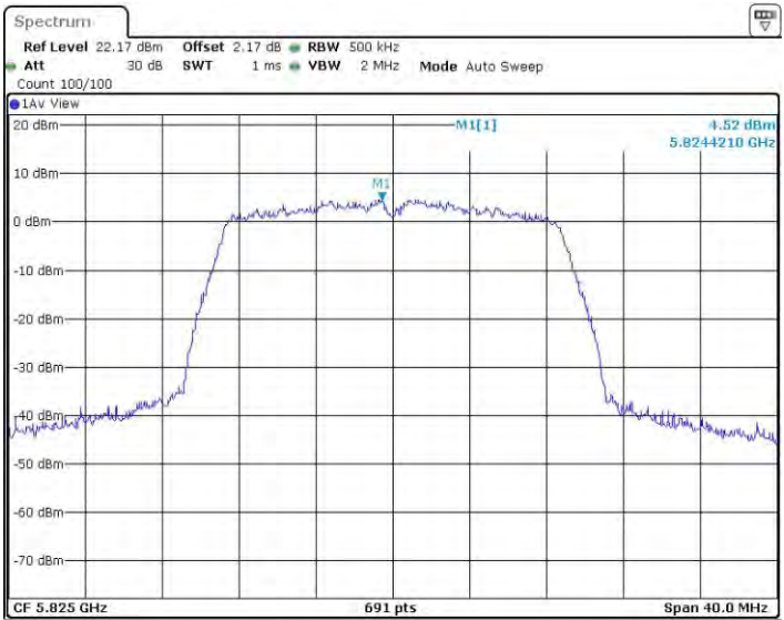
11N20MIMO_Ant4_5825
