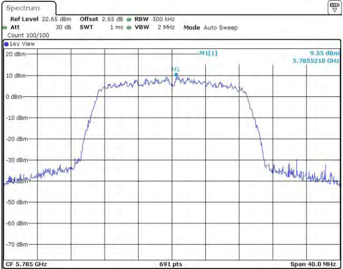
11AC20MIMO_Ant2_5785
