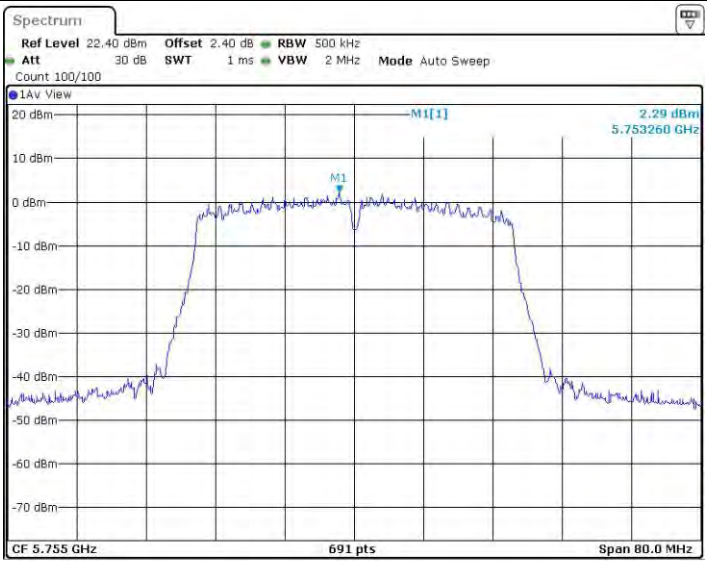
11N40BF_Ant1_5755
