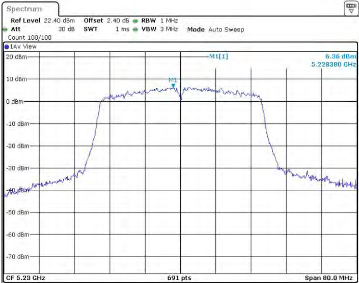
11N40MIMO_Ant4_5230
