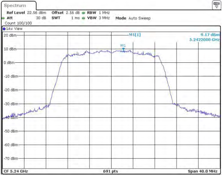
11N20MIMO_Ant3_5240
