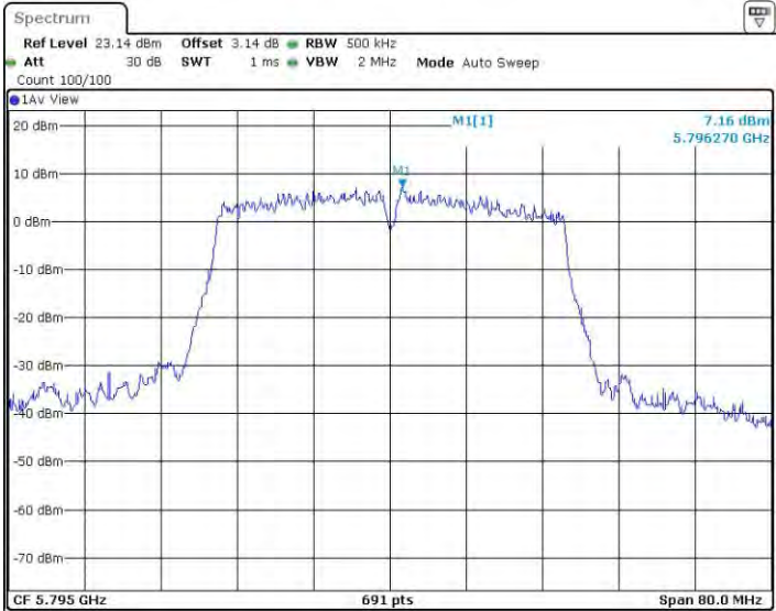
11AC40MIMO_Ant3_5795
