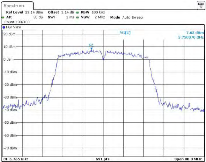
11AC40MIMO_Ant4_5755
