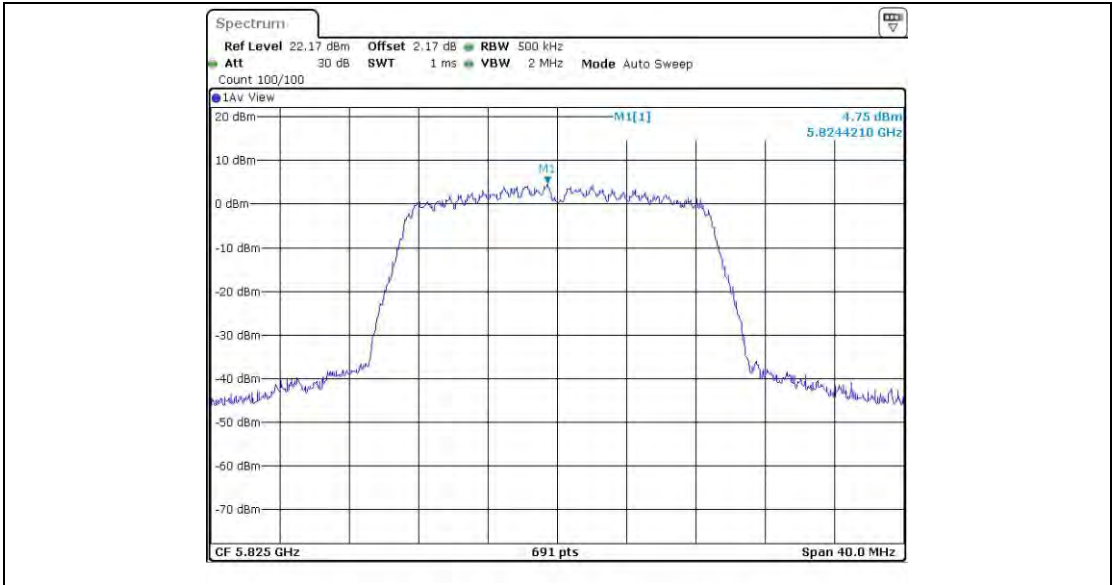
11N20BF_Ant2_5825
