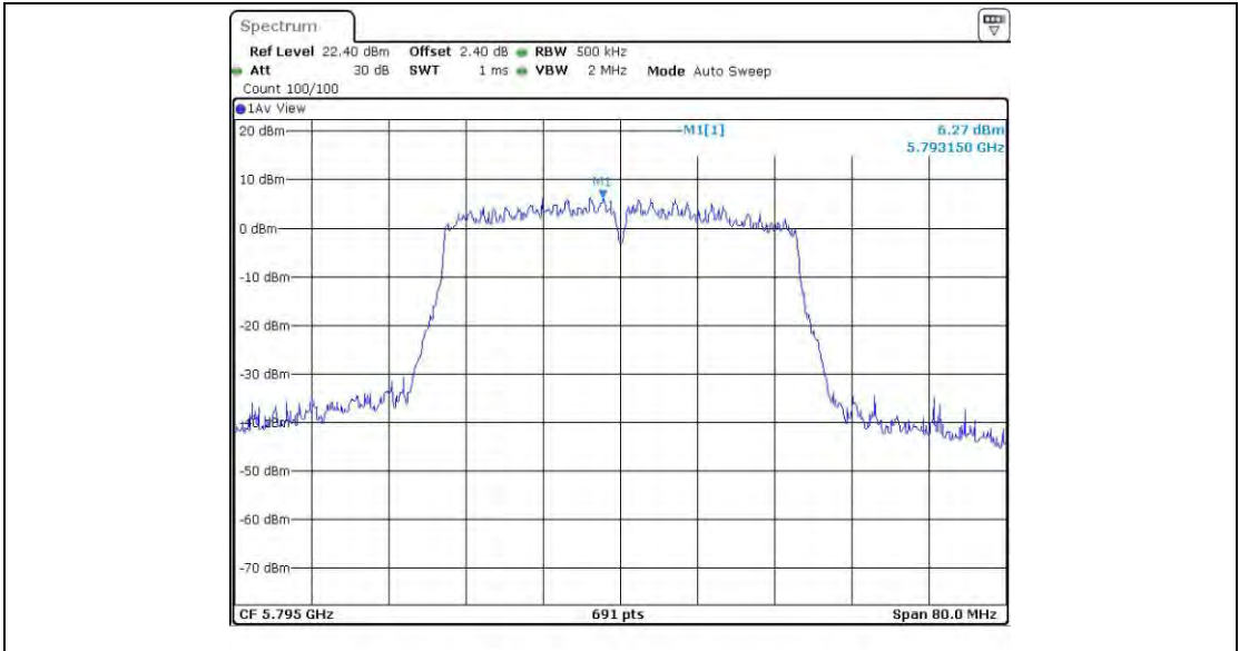
11N40MIMO_Ant3_5795
