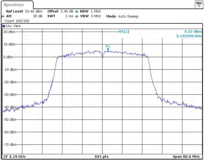
11N40MIMO_Ant4_5190
