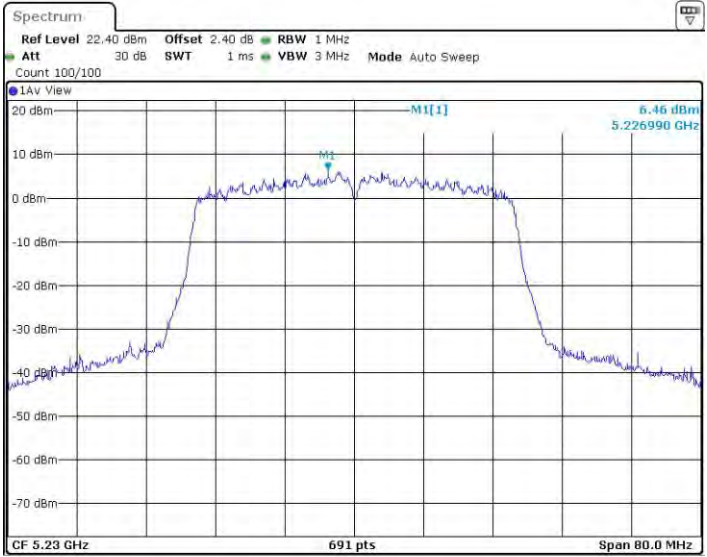
11N40BF_Ant1_5230
