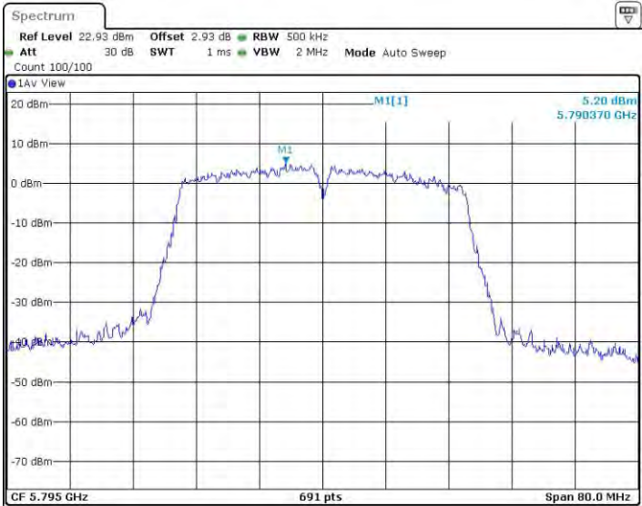
11AC40MIMO_Ant4_5795
