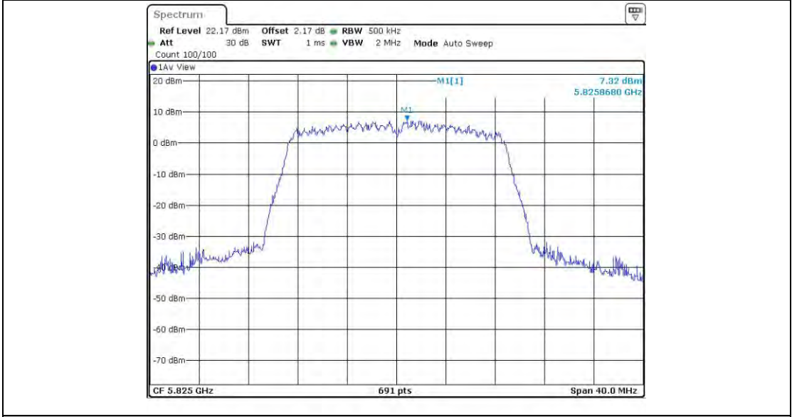
11N20MIMO_Ant3_5825
