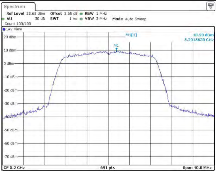
11AC20MIMO_Ant4_5200
