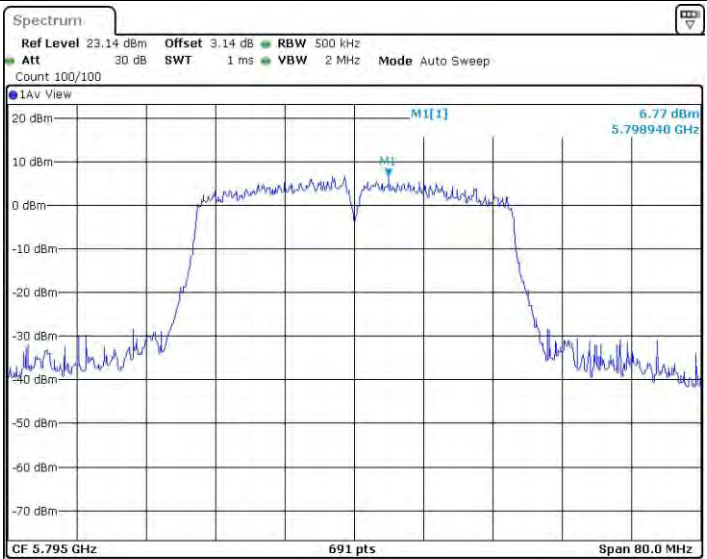
11AC40MIMO_Ant1_5795
