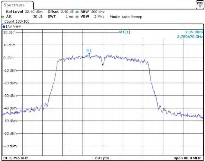
11N40SISO_Ant3_5795
