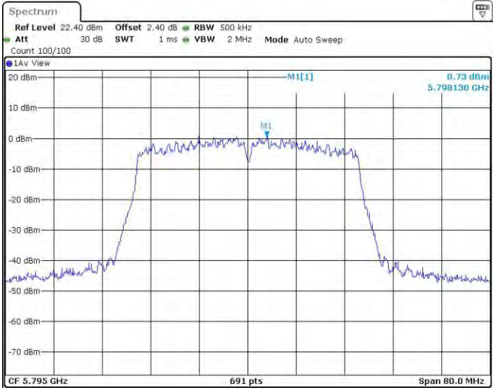
11N40BF_Ant2_5795
