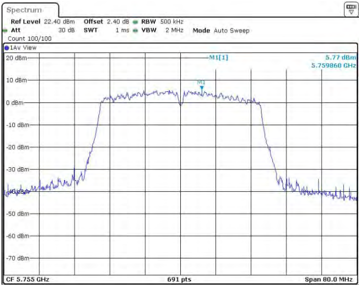
11N40MIMO_Ant4_5755
