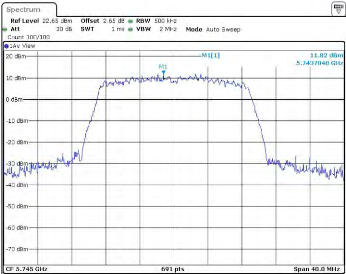
11AC20MIMO_Ant3_5745
