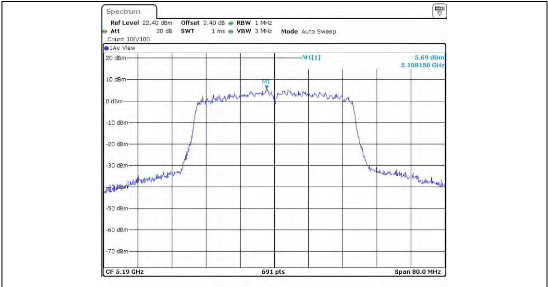
11N40BF_Ant1_5190
