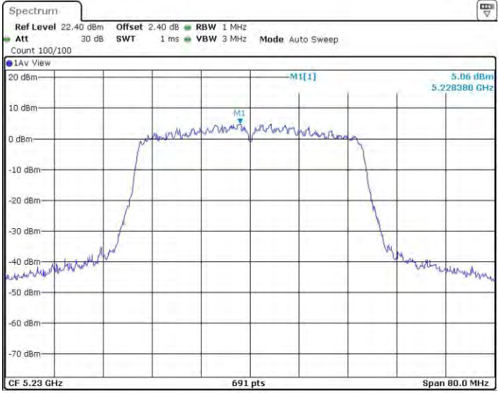
11N40BF_Ant2_5230
