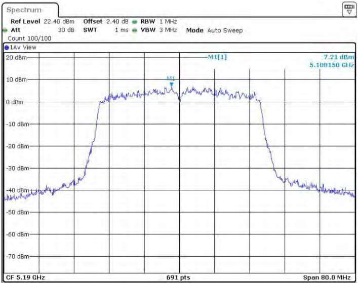
11N40MIMO_Ant3_5190
