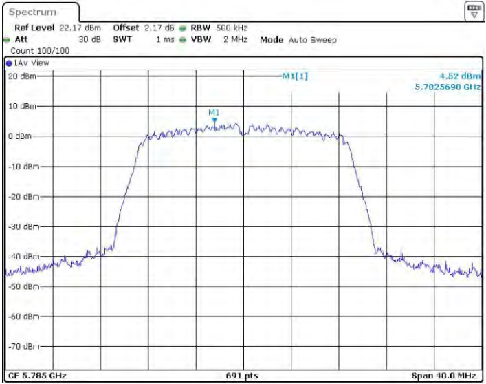
11N20BF_Ant2_5785
