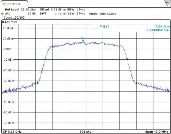
11AC20BF_Ant1_5180
