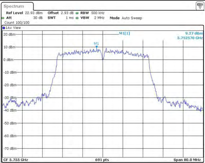
11AC40MIMO_Ant3_5755
