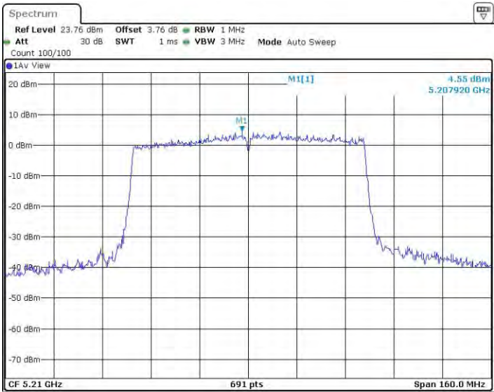
11AC80MIMO_Ant4_5210
