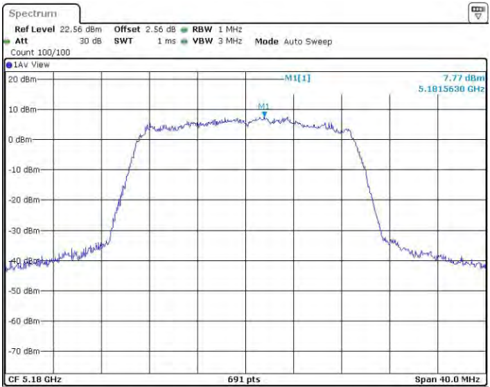
11N20MIMO_Ant3_5180
