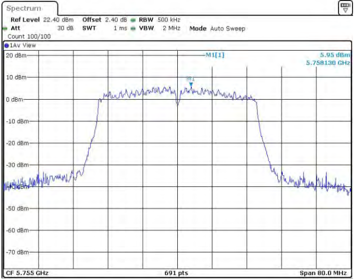
11N40MIMO_Ant2_5755
