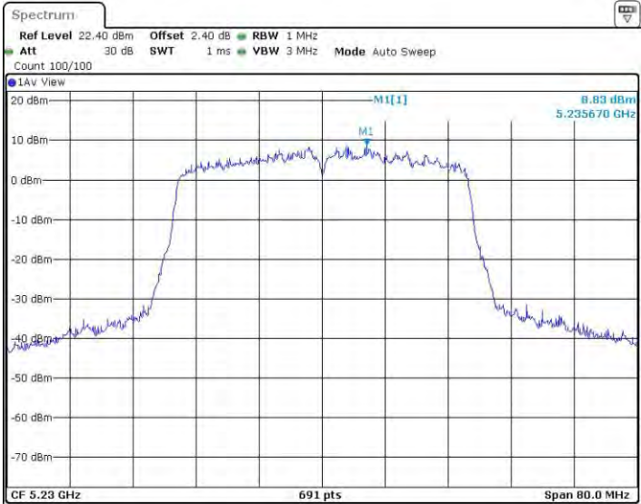
11N40MIMO_Ant3_5230
