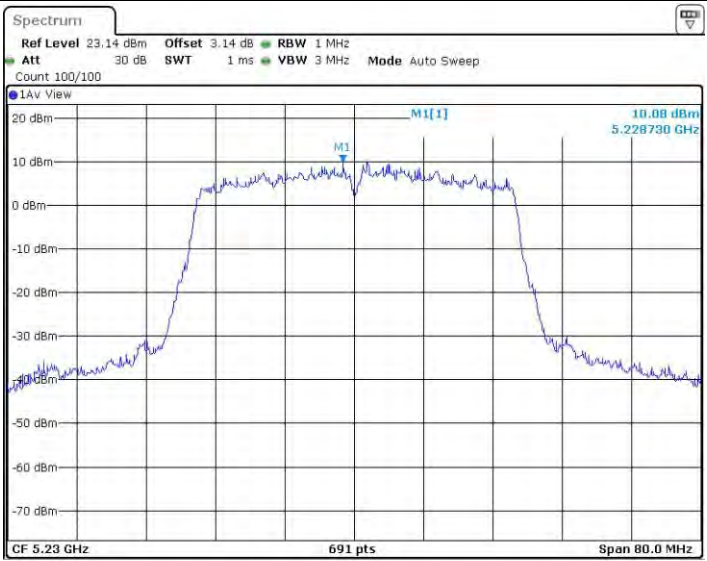
11AC40MIMO_Ant3_5230
