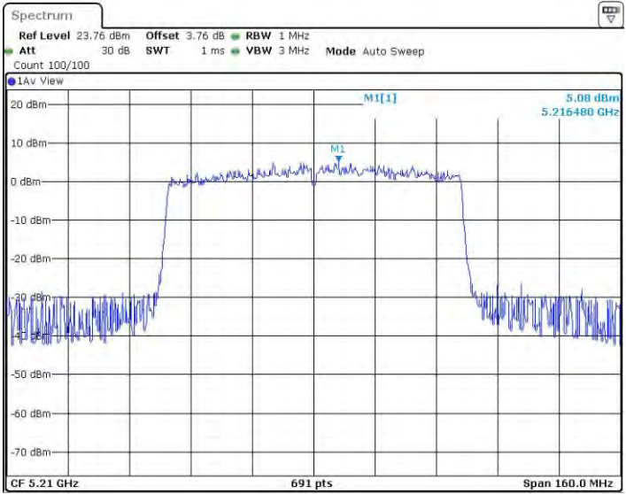
11AC80MIMO_Ant3_5210
