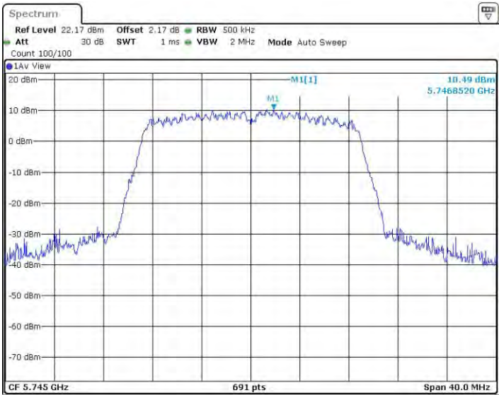
11N20MIMO_Ant3_5745
