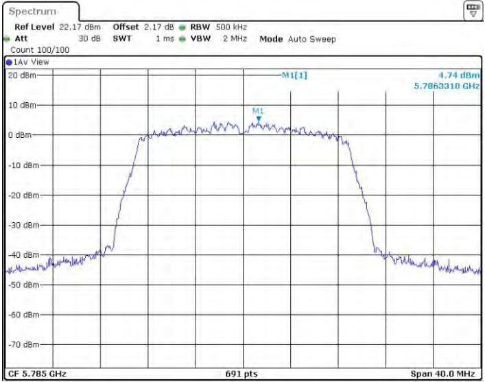
11N20BF_Ant1_5785
