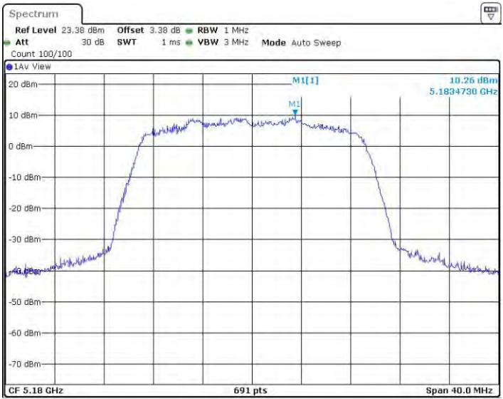
11AC20MIMO_Ant3_5180
