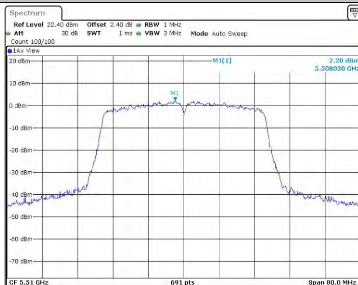
11N40SISO_Ant3_5510
