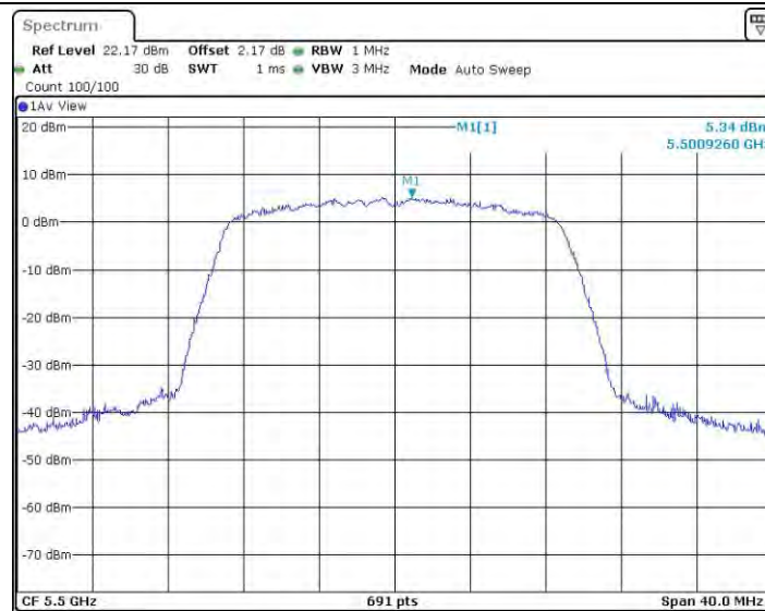
11N20SISO_Ant4_5500
