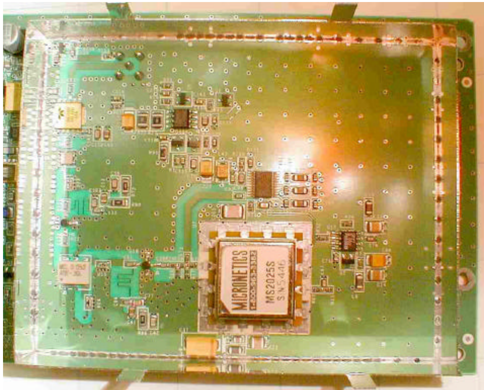
RFC Bottom Right
