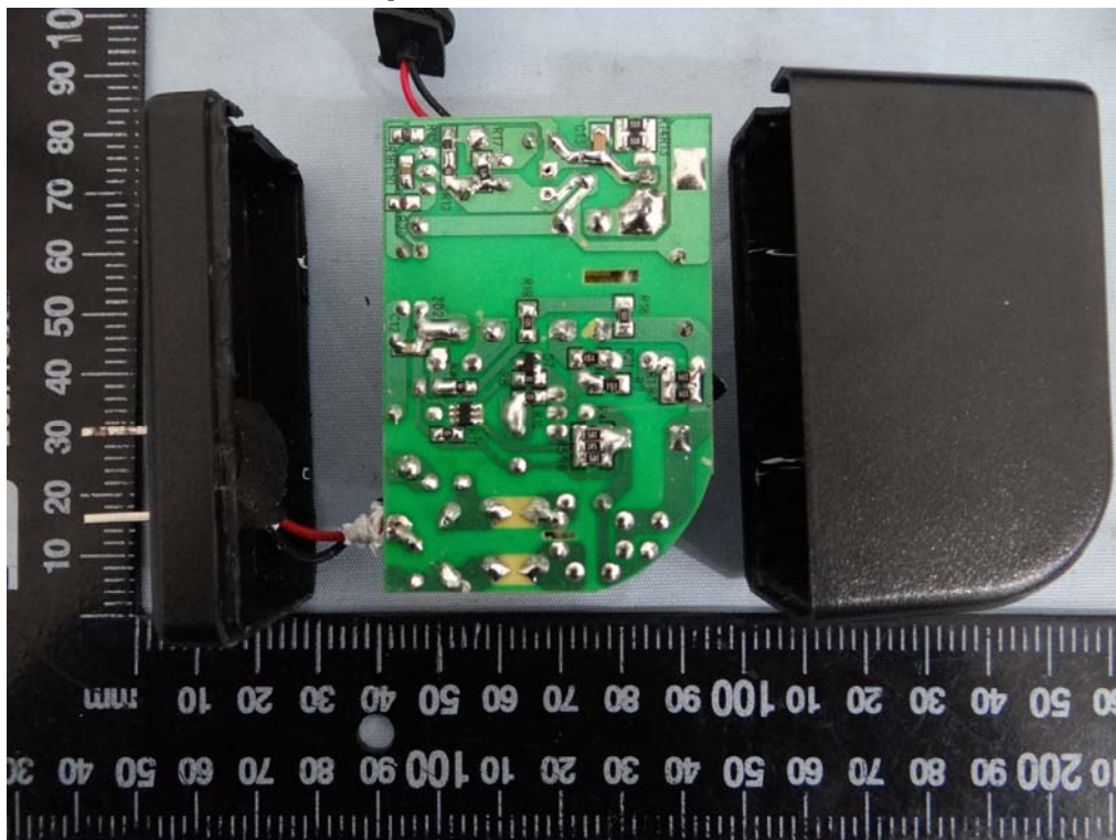
Adapter 2 (SAW24-180-1300)
