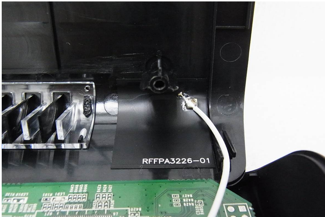
EUT 6 Antenna 2
