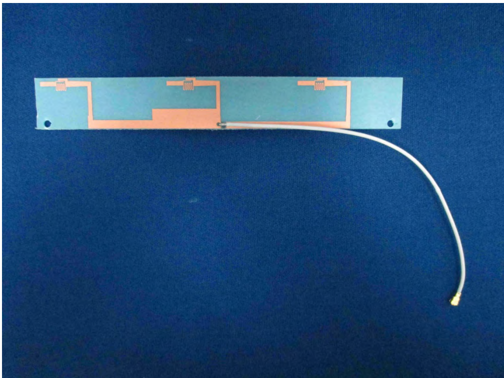
(8) EUT Photo (ANT0)
