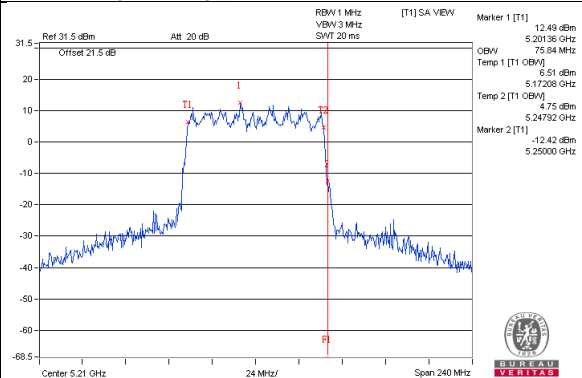
802.11ac(VHT80)_Chain4 / CH42
