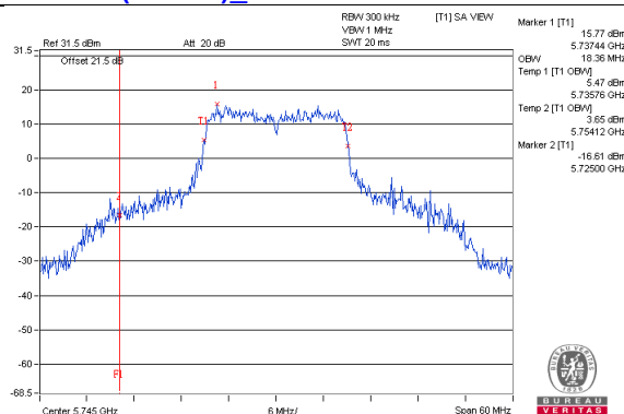
802.11ac(VHT20)_Chain3 / CH149
