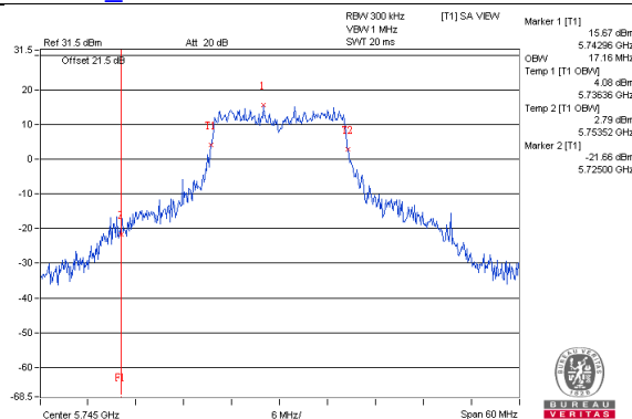
802.11a_Chain3 / CH149
