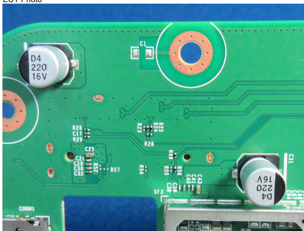
(36) EUT Photo
