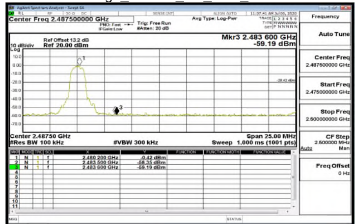
Band Edge 8DPSK 3M DH5 2480MHz
