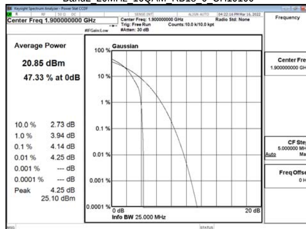
Band2 20MHz 16QAM RB18 0 CH19100
