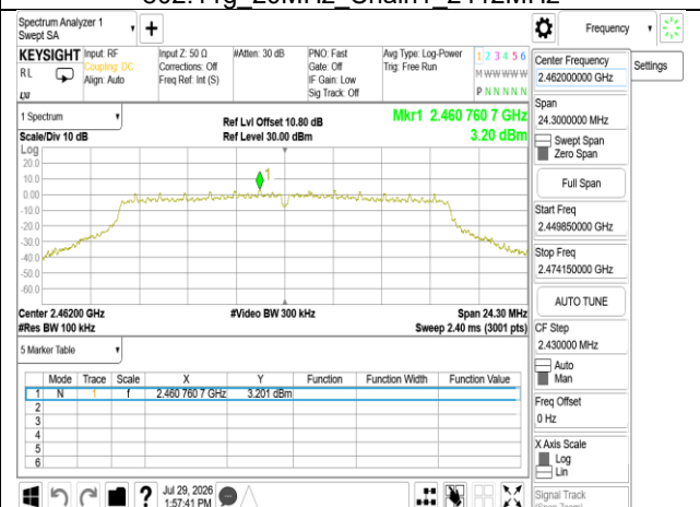
802.11g_20MHz_Chain1_2462MHz
