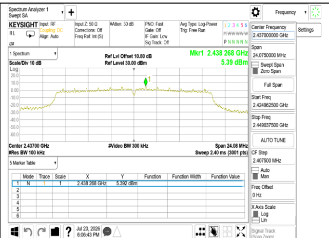
802.11g_20MHz_Chain0_2437MHz
