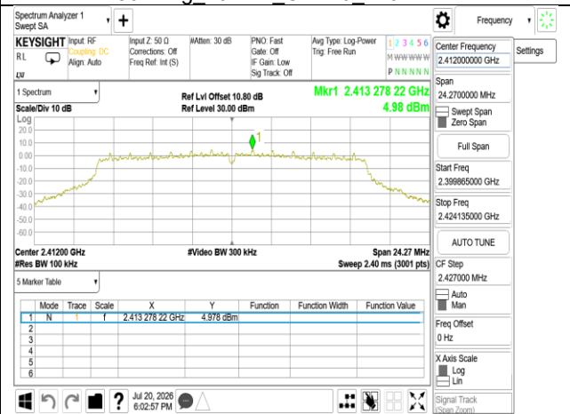
802.11g_20MHz_Chain1_2412MHz
