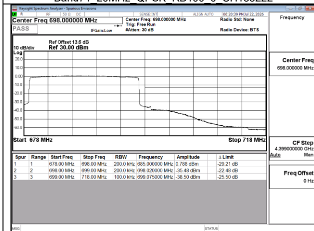
Band71 20MHz QPSK RB100 0 CH133372
