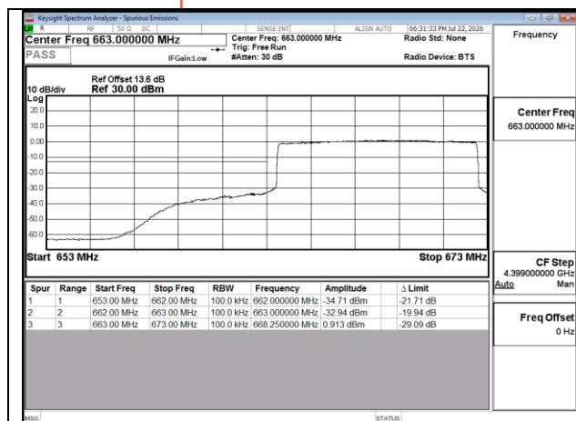
Band71 10MHz QPSK RB50 0 CH133172
