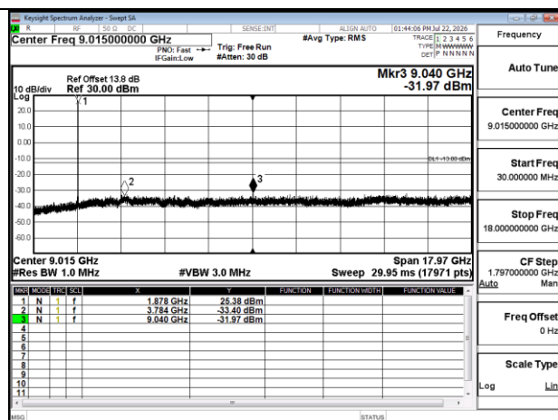
Band2 5MHz QPSK RB1 0 CH18900 below 18G
