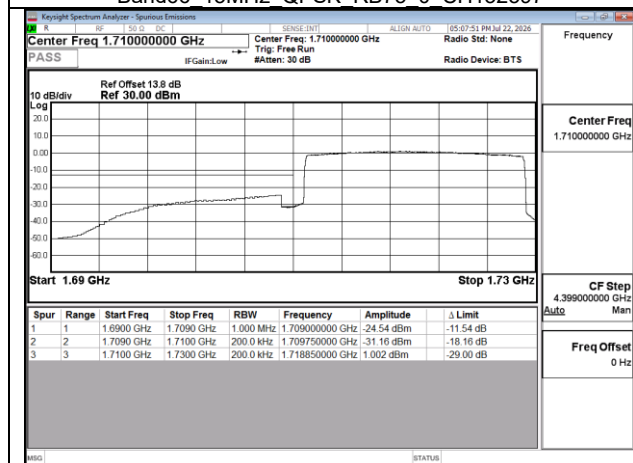
Band66 20MHz QPSK RB100 0 CH132072
