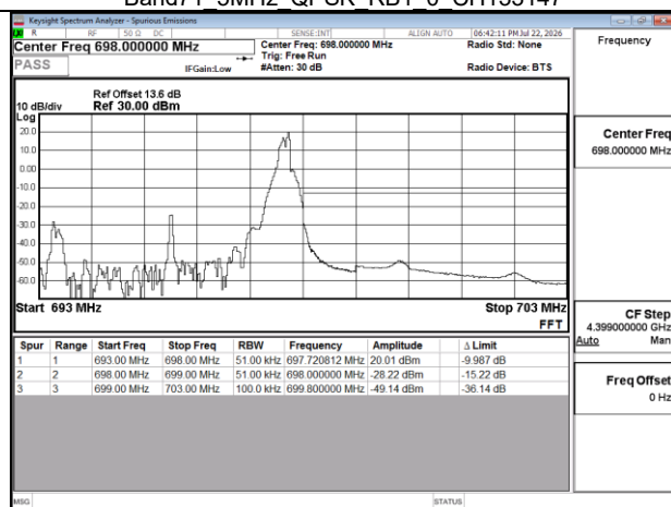
Band71 5MHz QPSK RB1 24 CH133447
