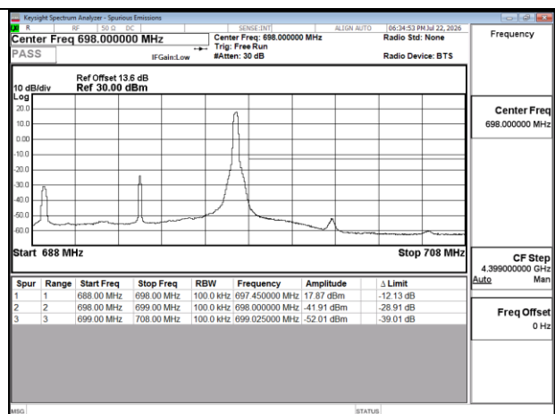
Band71 10MHz QPSK RB1 49 CH133422
