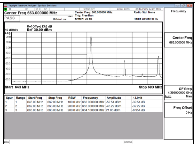
Band71 20MHz QPSK RB1 0 CH133222
