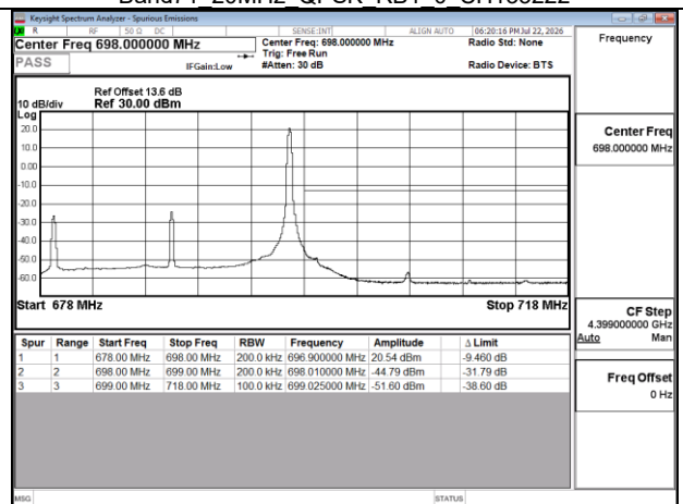
Band71 20MHz QPSK RB1 99 CH133372
