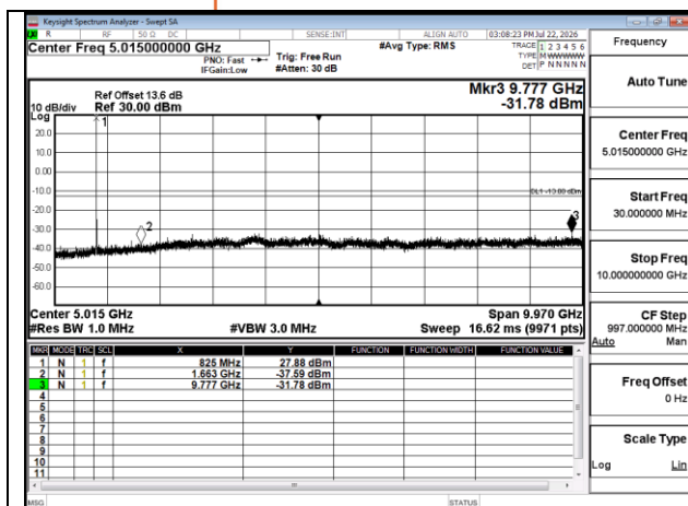
Band5 5MHz QPSK RB1 0 CH20425 below 18G
