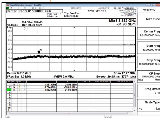
Band2 5MHz QPSK RB1 0 CH18625 below 18G
