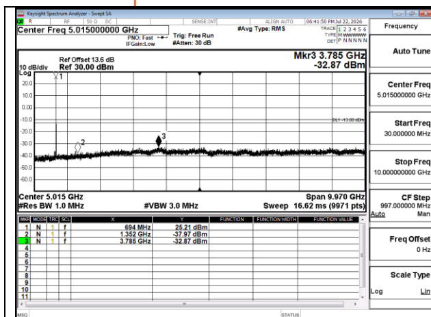
Band71 5MHz QPSK RB1 0 CH133447 below 18G
