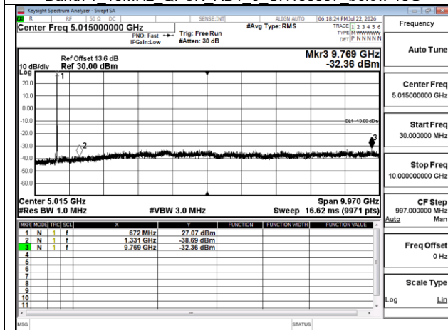
Band71 20MHz QPSK RB1 0 CH133297 below 18G
