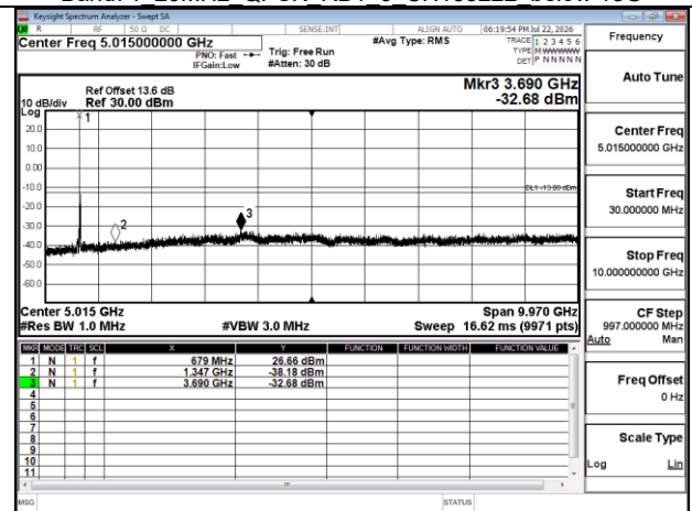
Band71 20MHz QPSK RB1 0 CH133372 below 18G
