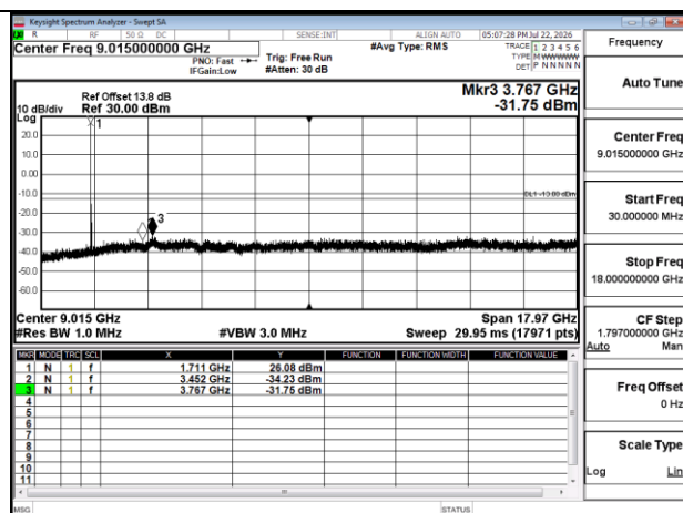
Band66 20MHz QPSK RB1 0 CH132072 below 18G
