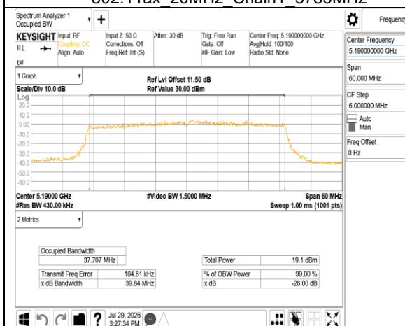
802.11ax 40MHz Chain0 5190MHz
