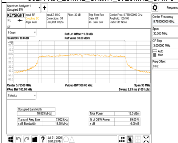
802.11ax 20MHz Chain1 5785MHz
