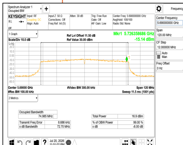
802.11ac 80MHz Chain1 5690MHz UNII-3
