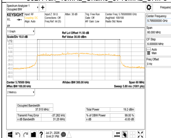
802.11ax 40MHz Chain0 5795MHz
