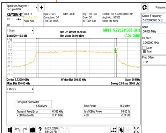
802.11ax 20MHz Chain1 5720MHz UNII-3
