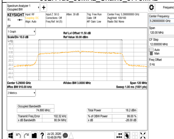
802.11ac 80MHz Chain1 5290MHz
