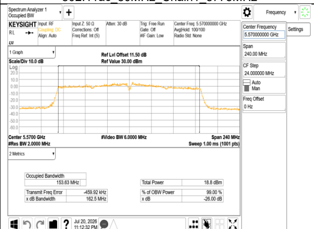
802.11ac 160MHz Chain0 5570MHz
