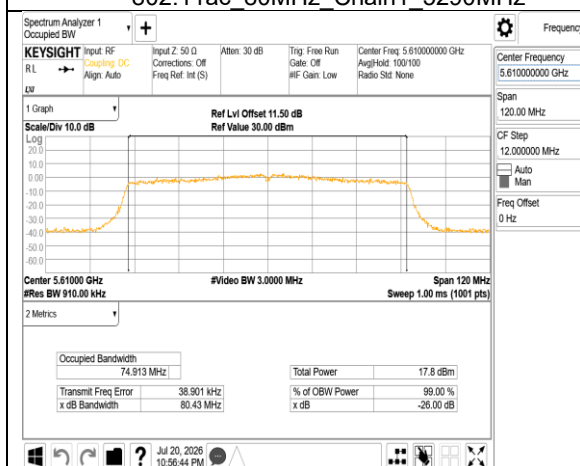
802.11ac 80MHz Chain1 5610MHz
