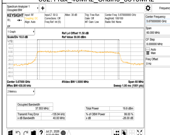
802.11ax 40MHz Chain0 5670MHz
