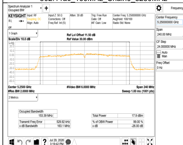
802.11ac 160MHz Chain1 5250MHz
