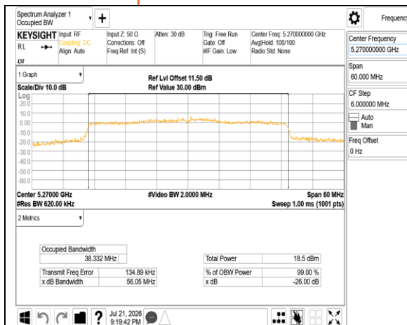
802.11ax 40MHz Chain0 5270MHz
