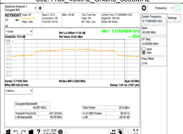
802.11ax 40MHz Chain0 5710MHz UNII-2C
