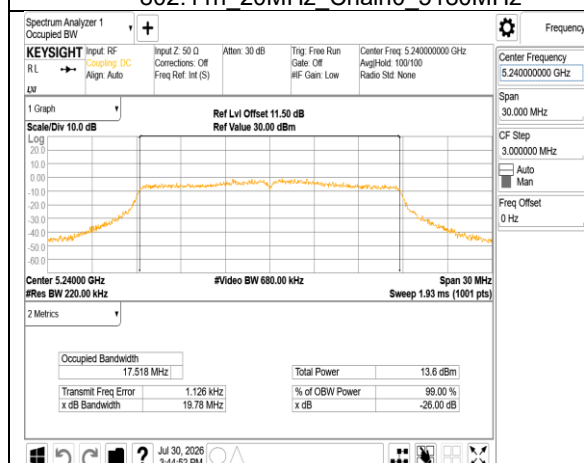
802.11n_20MHz_Chain0_5240MHz
