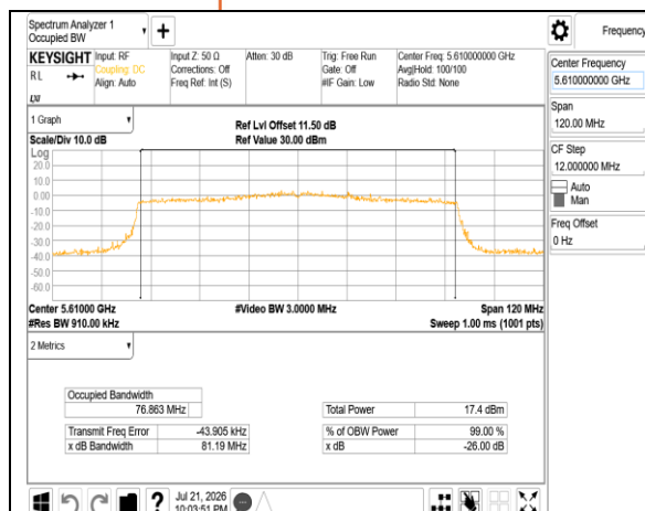
802.11ax_80MHz_Chain1_5610MHz
