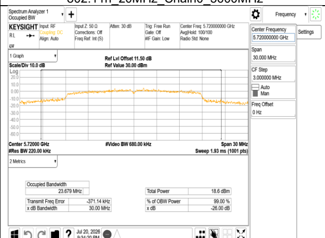
802.11n 20MHz Chain0 5720MHz
