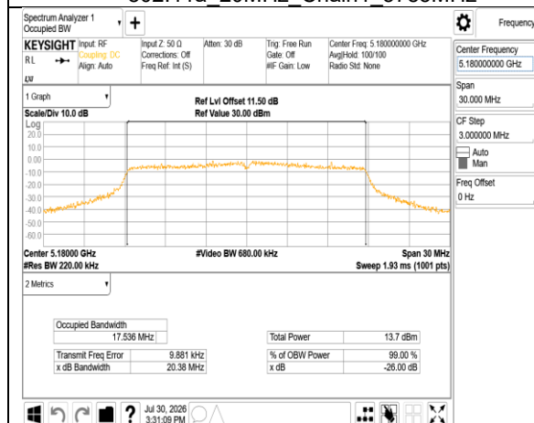
802.11n_20MHz_Chain0_5180MHz
