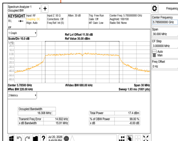
802.11a_20MHz_Chain1_5785MHz
