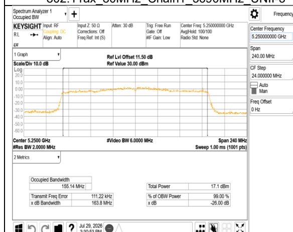
802.11ax_160MHz_Chain0_5250MHz
