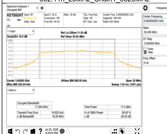
802.11n 20MHz Chain1 5600MHz
