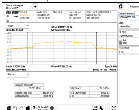
802.11a_20MHz_Chain0_5500MHz
