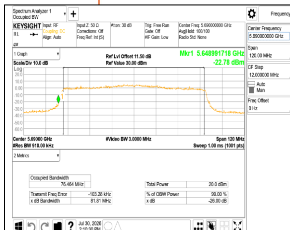
802.11ax 80MHz Chain0 5690MHz UNII-2C
