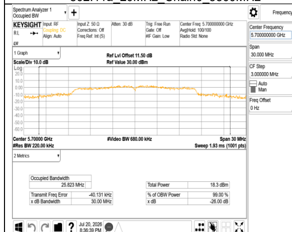
802.11a_20MHz_Chain0_5700MHz
