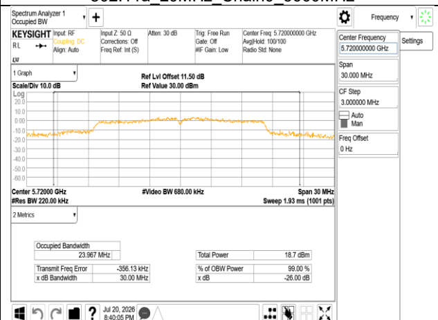
802.11a_20MHz_Chain0_5720MHz
