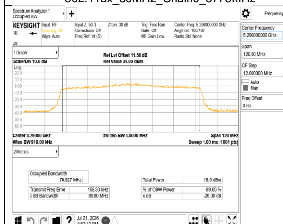
802.11ax 80MHz Chain1 5290MHz
