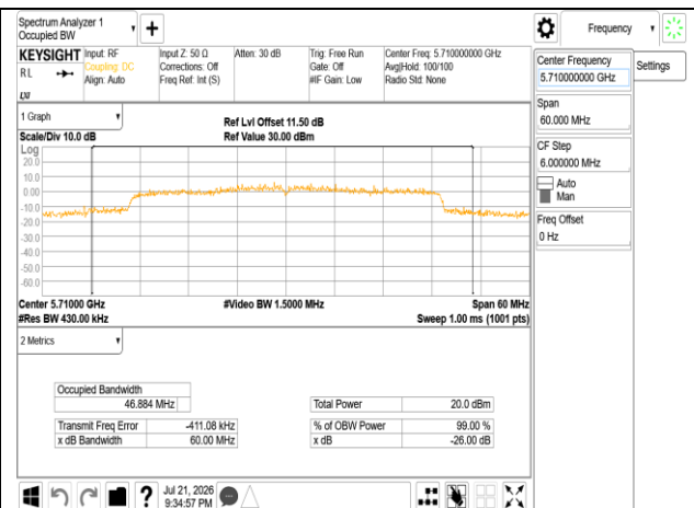
802.11ax 40MHz Chain0 5710MHz
