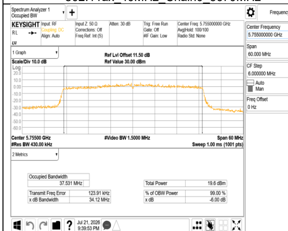
802.11ax 40MHz Chain0 5755MHz
