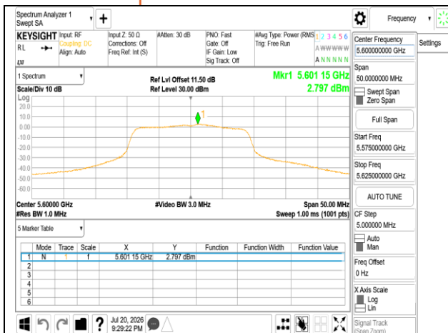
802.11n 20MHz Chain0_5600MHz
