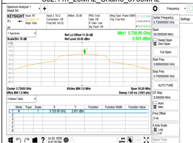
802.11n 20MHz Chain0_5720MHz UNII 2C
