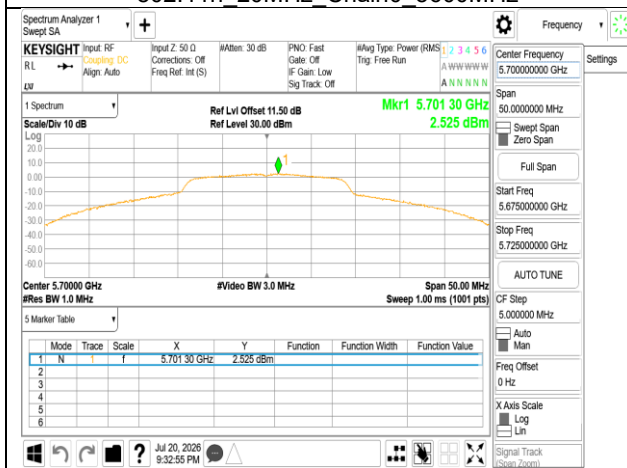
802.11n 20MHz Chain0_5700MHz
