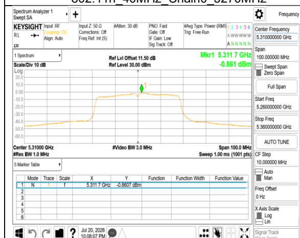
802.11n 40MHz Chain0_ 5310MHz
