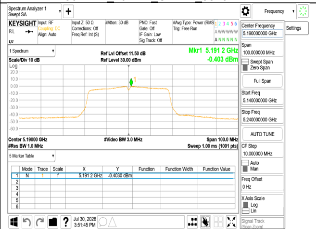
802.11n_40MHz_Chain1_5190MHz
