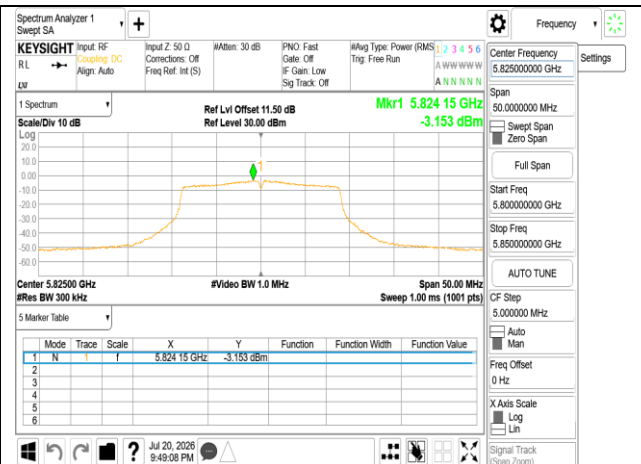
802.11n_20MHz_Chain1_5825MHz
