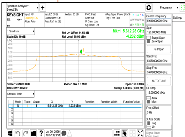
802.11ac 80MHz Chain0 5610MHz
