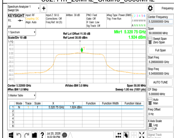
802.11n 20MHz Chain0_5320MHz
