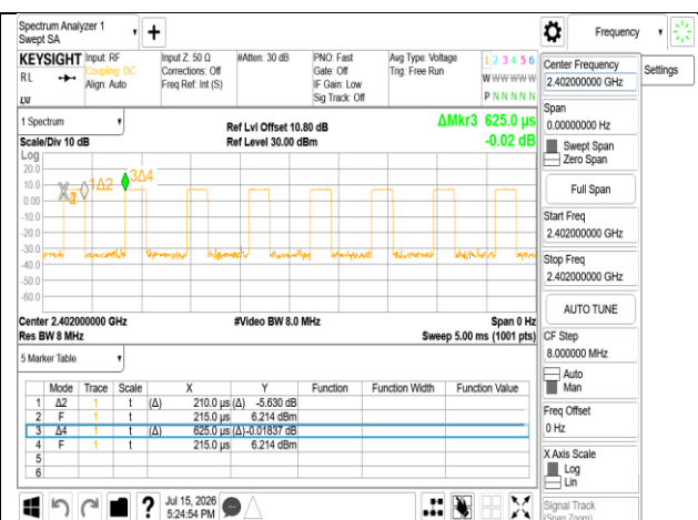
BLE 2M 2402MHz
