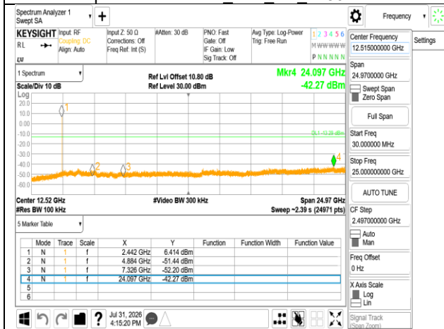
Spurious Emission BLE 2M 2442MHz
