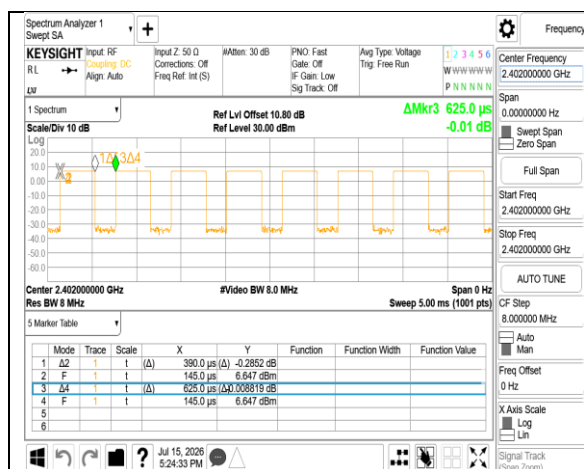
BLE 1M 2402MHz
