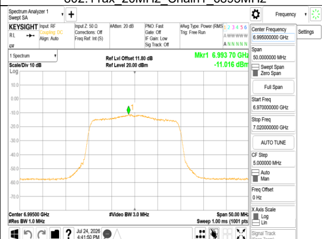
802.11ax 20MHz Chain1 6995MHz
