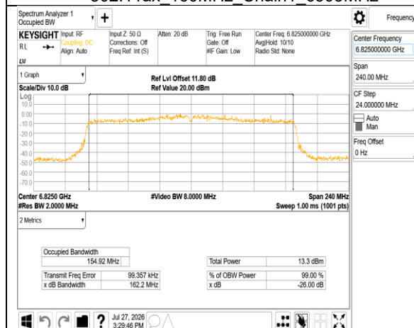
802.11ax 160MHz Chain1 6825MHz
