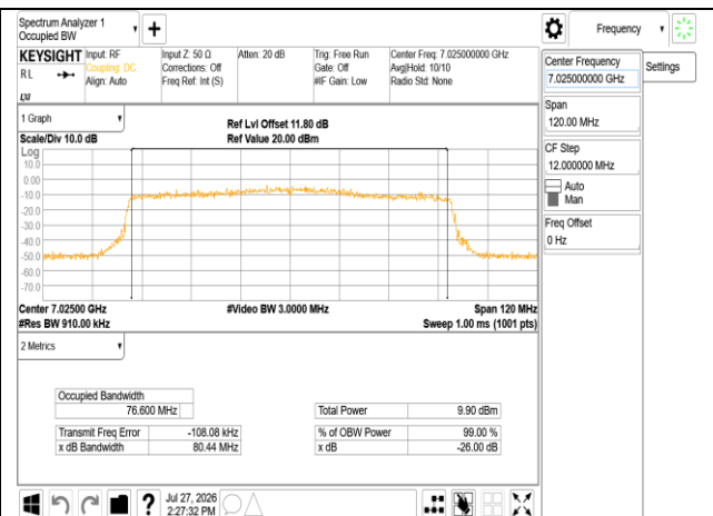
802.11ax_80MHz_Chain1_7025MHz
