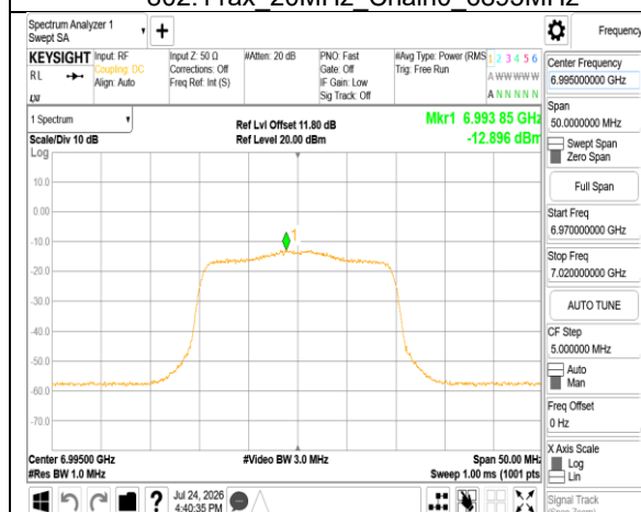
802.11ax 20MHz Chain0 6995MHz
