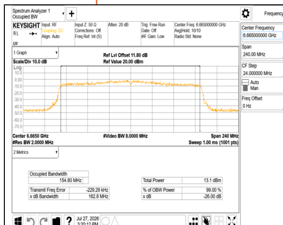
802.11ax_160MHz_Chain0_6665MHz
