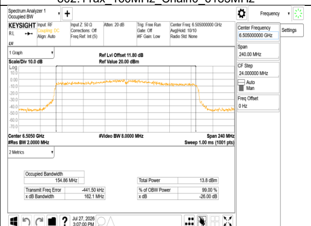
802.11ax_160MHz_Chain0_6505MHz
