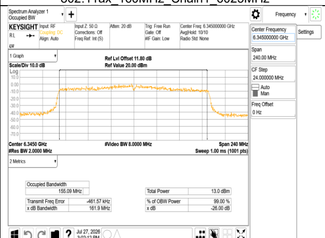
802.11ax_160MHz_Chain1_6345MHz
