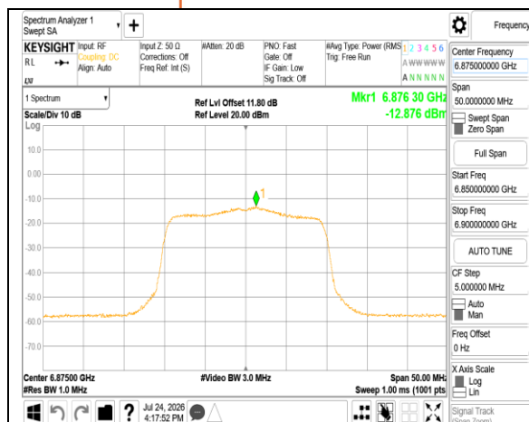
802.11ax 20MHz Chain0 6875MHz
