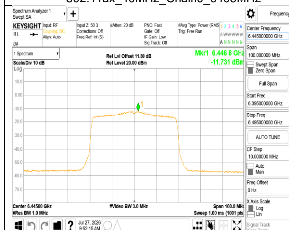
802.11ax 40MHz Chain0 6445MHz
