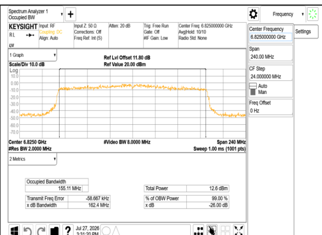
802.11ax_160MHz_Chain0_6825MHz
