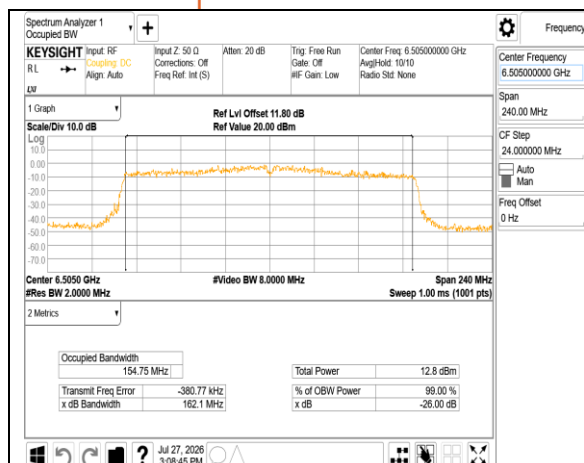
802.11ax 160MHz Chain1 6505MHz
