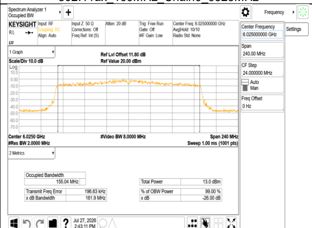
802.11ax_160MHz_Chain1_6025MHz
