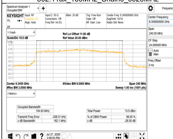
802.11ax_160MHz_Chain0_6345MHz
