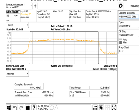
802.11ax_160MHz_Chain0_6985MHz
