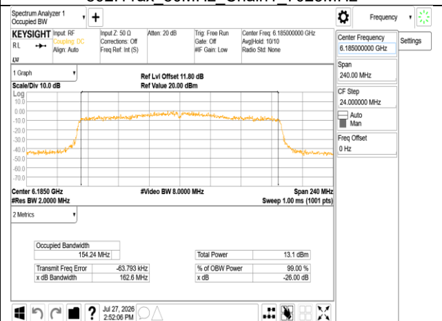
802.11ax_160MHz_Chain0_6185MHz
