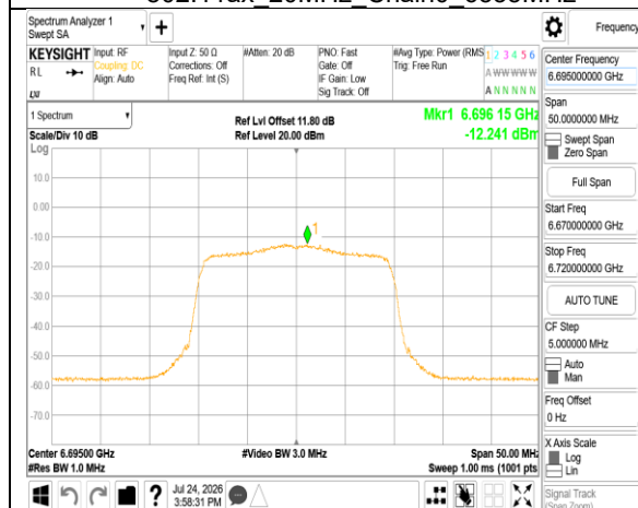
802.11ax 20MHz Chain0 6695MHz
