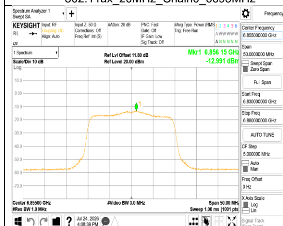
802.11ax 20MHz Chain0 6855MHz
