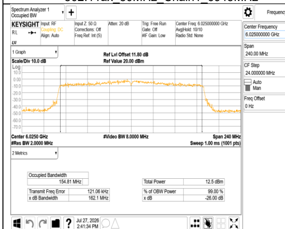
802.11ax_160MHz_Chain0_6025MHz
