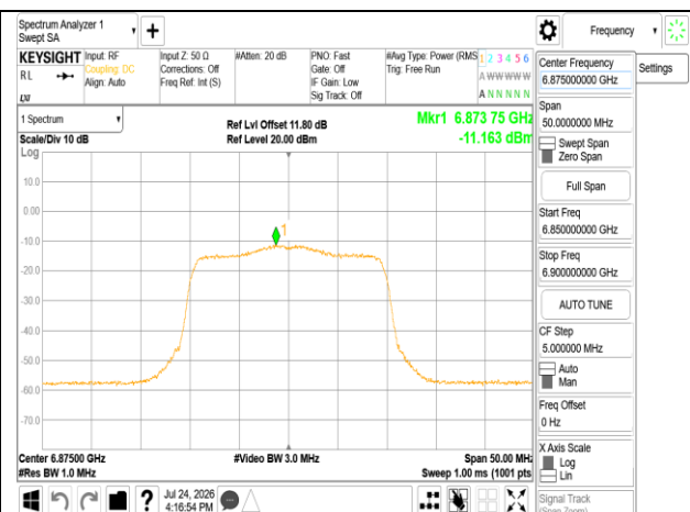
802.11ax 20MHz Chain1 6875MHz
