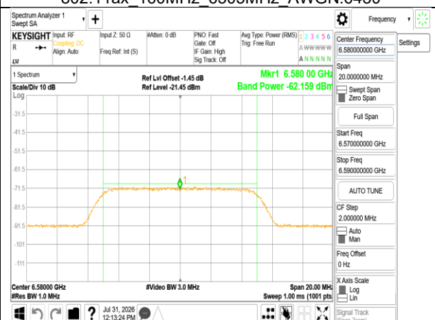
802.11ax 160MHz 6505MHz AWGN:6580
