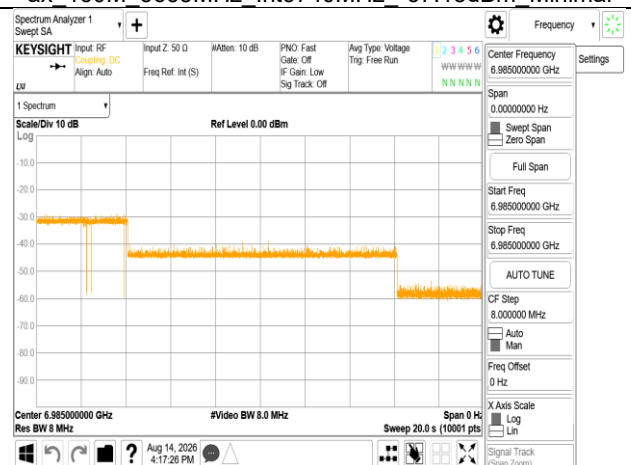
ax 160M 6985MHz Int6910MHz -62.10dBm OFF
