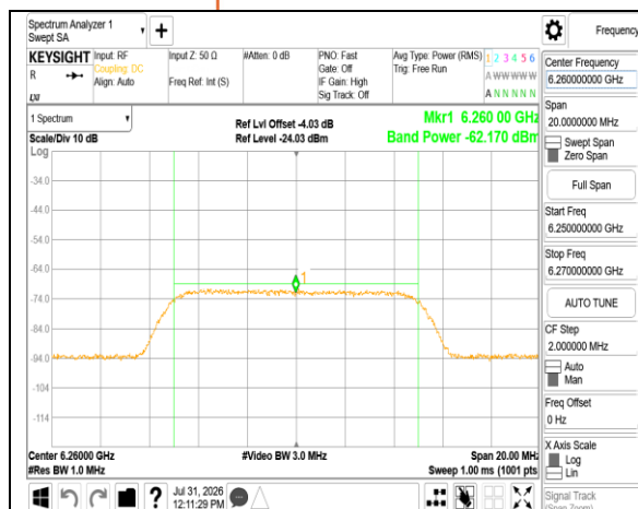
802.11ax 160MHz 6185MHz AWGN:6260
