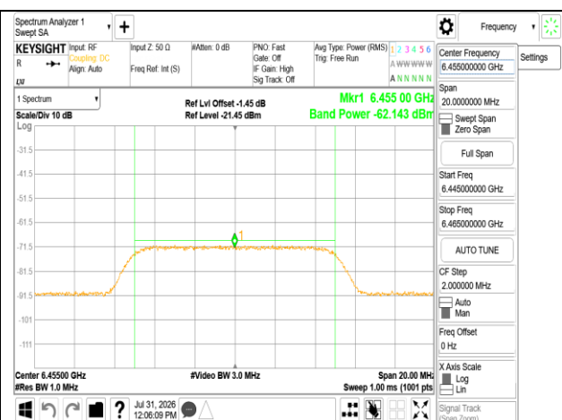
802.11ax 20MHz 6455MHz AWGN:6455MHz
