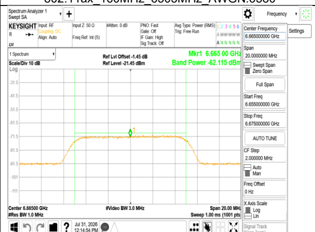
802.11ax 160MHz 6665MHz AWGN:6665MHz
