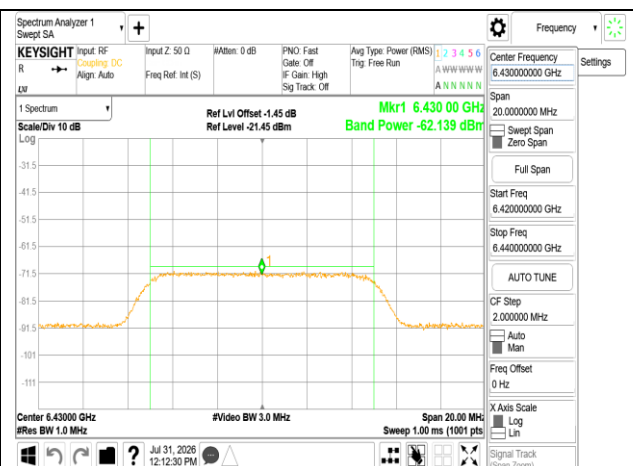
802.11ax 160MHz 6505MHz AWGN:6430
