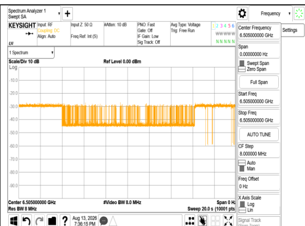
ax 160M 6505MHz Int6505MHz -63.13dBm Minimal
