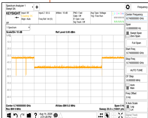
ax 160M 6665MHz Int6740MHz -65.15dBm OFF
