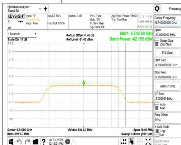
802.11ax 160MHz 6665MHz AWGN:6740
