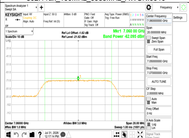
802.11ax 160MHz 6985MHz AWGN:7060
