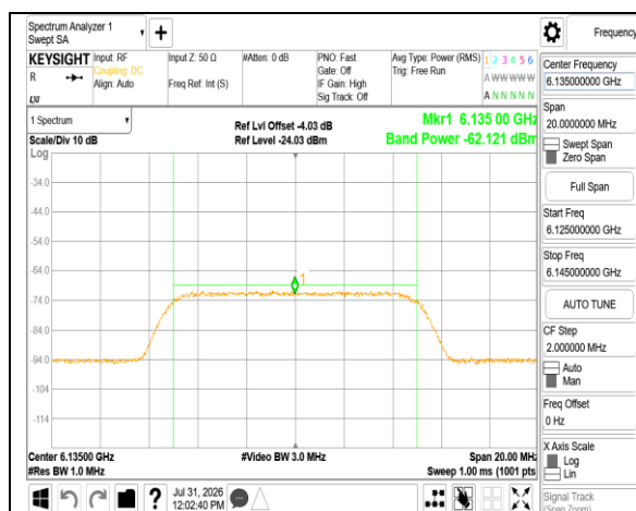
802.11ax 20MHz 6135MHz AWGN:6135MHz
