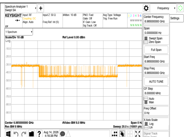
ax 160M 6985MHz Int6985MHz -63.10dBm Minimal
