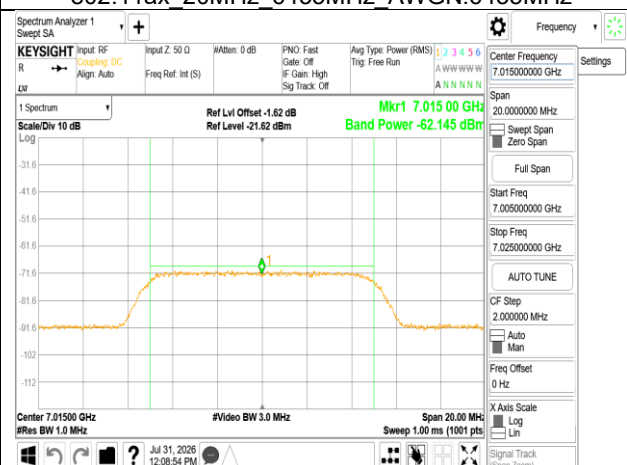
802.11ax 20MHz 7015MHz AWGN:7015MHz
