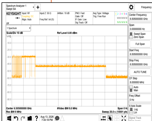
ax 160M 6505MHz Int6505MHz -62.13dBm OFF
