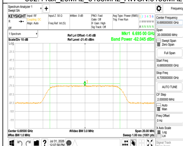
802.11ax 20MHz 6695MHz AWGN:6695MHz
