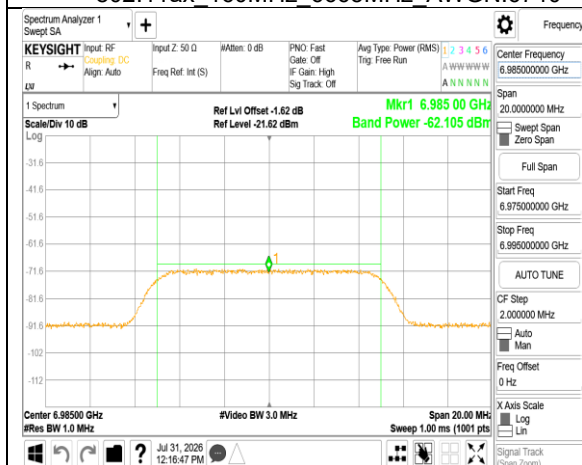
802.11ax 160MHz 6985MHz AWGN:6985MHz
