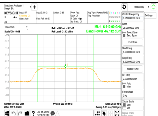
802.11ax 160MHz 6985MHz AWGN:6910
