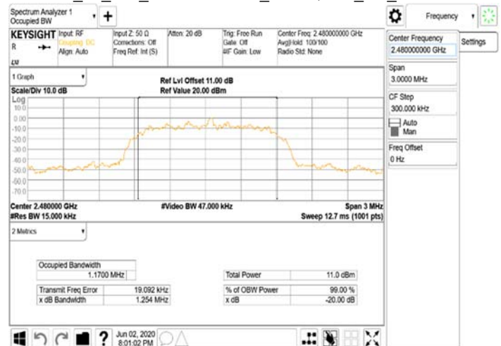
FCC_15_247_BT\OBW 20dB \pi/4 DQPSK_2M_2480MHz
