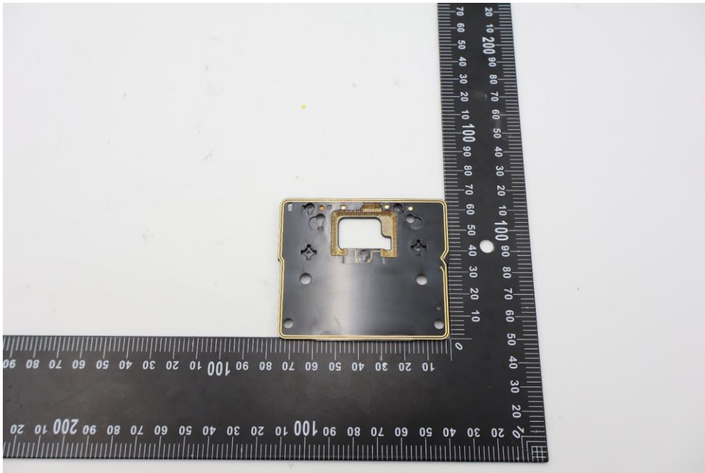
NFC Antenna
