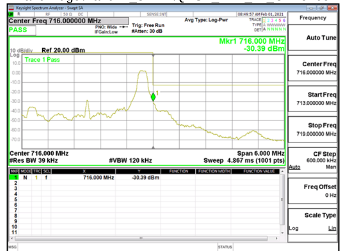
Band Edge\Band12_3MHz\QPSK_RB1_14_CH23165
