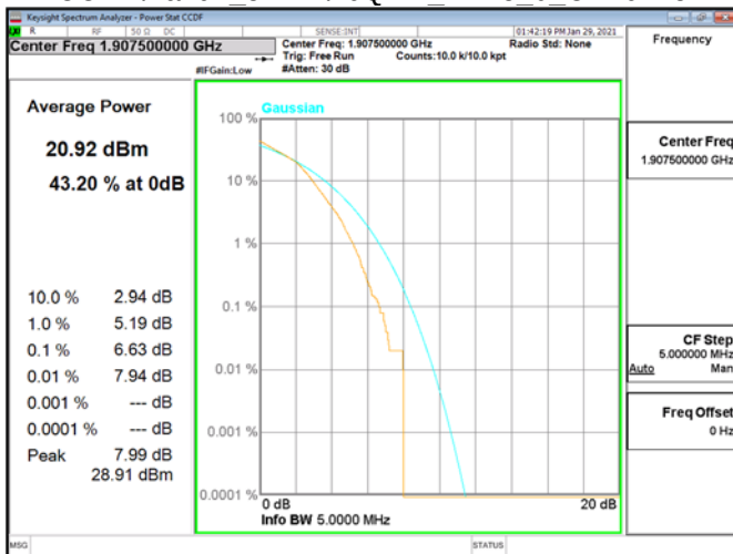
CCDF\Band2 5MHz\16QAM RB25 0 CH19175
