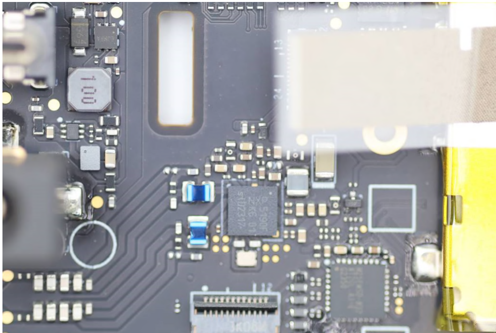
NFC RFIC
