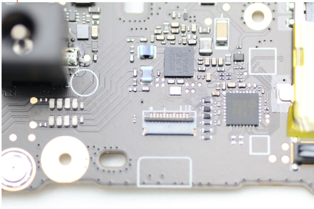
NFC Antenna-1
