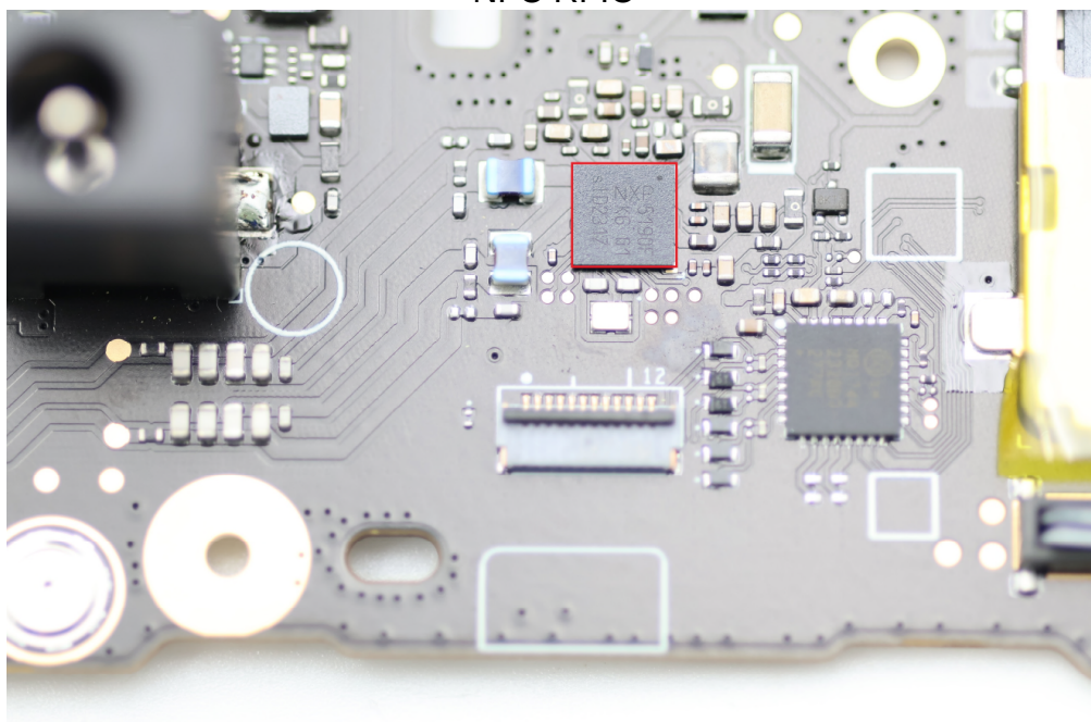
NFC RFIC
