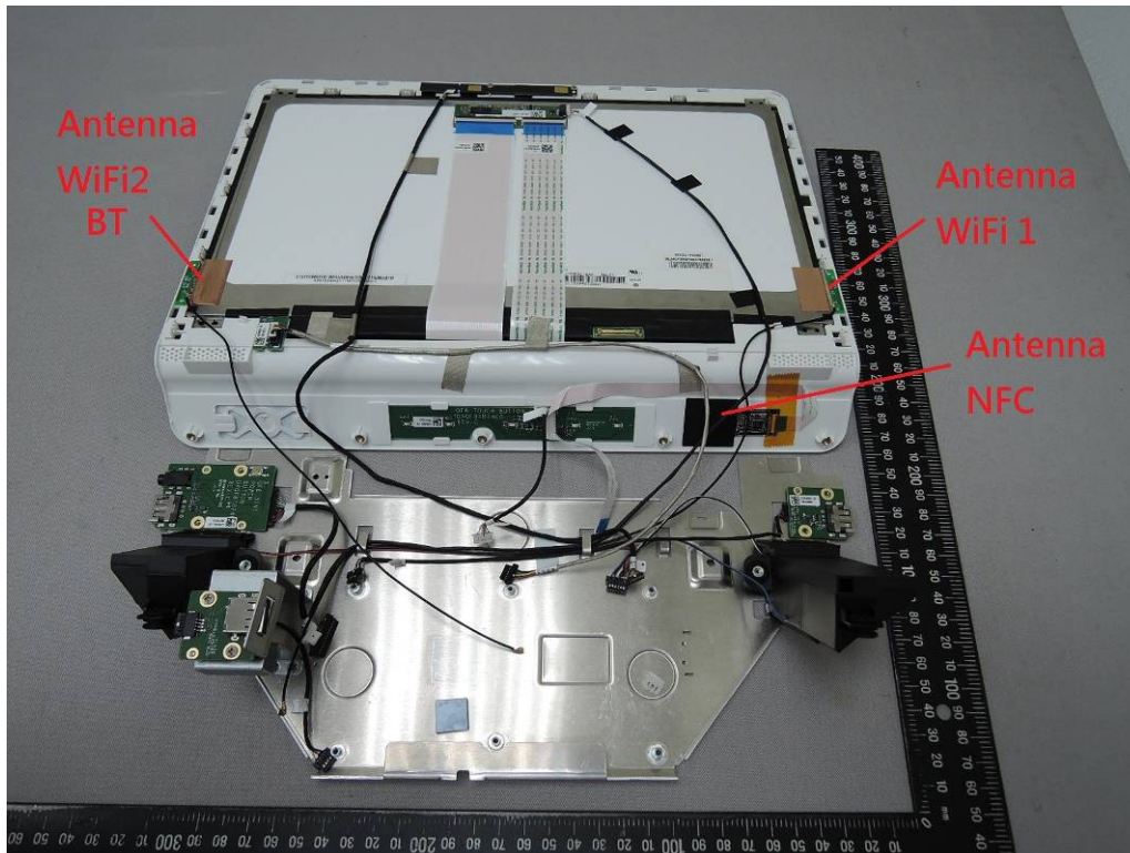
BT / WLAN / NFC Antenna
