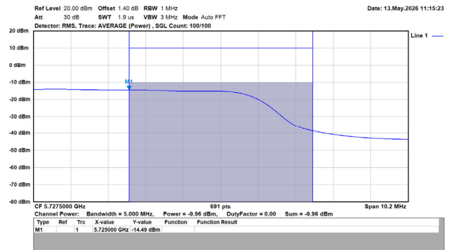
802.11ac/40MHz/MCS0/5710MHz/Ch142/Ant.2 (UNII-3)
