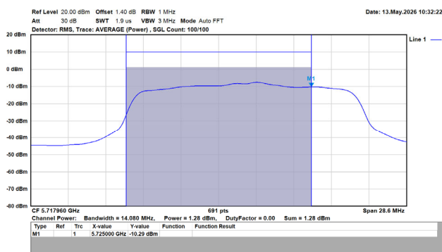
802.11a/20MHz/6M/5720MHz/Ch144/Ant.2 (UNII-2C)
