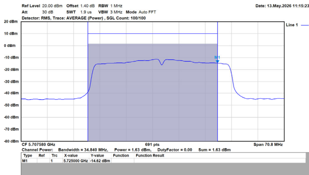
802.11ac/40MHz/MCS0/5710MHz/Ch142/Ant.2 (UNII-2C)
