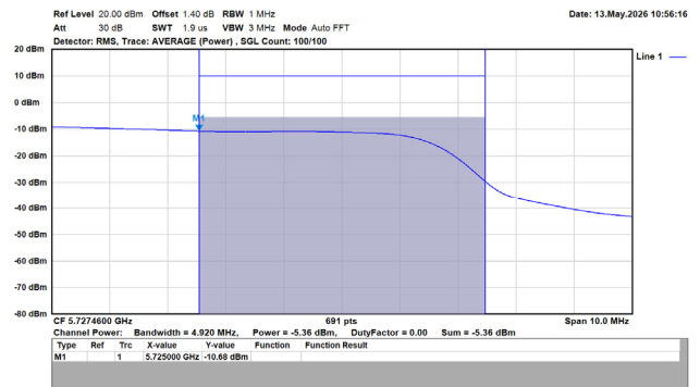
802.11ac/40MHz/MCS0/5710MHz/Ch142/Ant.1 (UNII-3)
