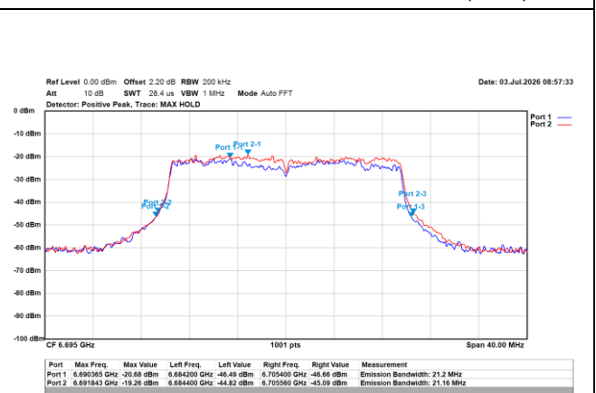
802.11ax/20MHz/MCS0/6695MHz/Ch149 (EBW)
