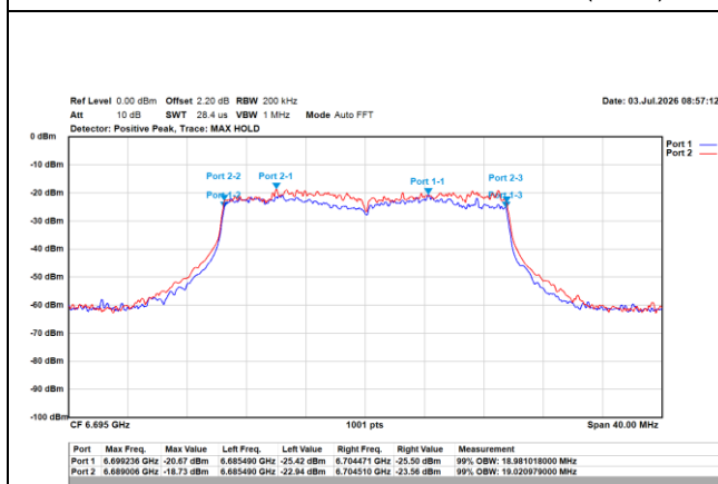
802.11ax/20MHz/MCS0/6695MHz/Ch149 (OBW)
