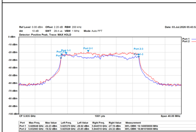
802.11ax/20MHz/MCS0/5935MHz/Ch2 (OBW)
