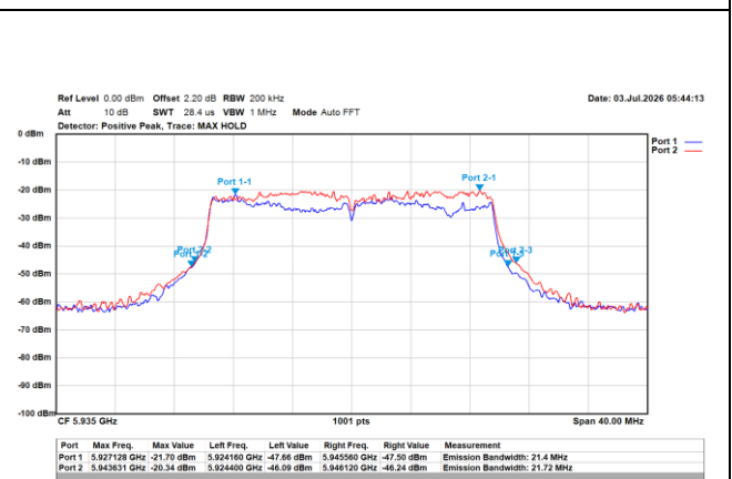
802.11ax/20MHz/MCS0/5935MHz/Ch2 (EBW)
