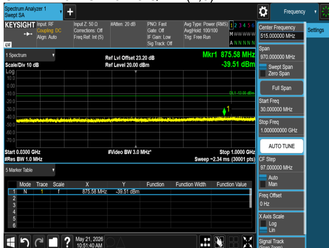
CSE B4 20M CH20300 QPSK(1,0)
