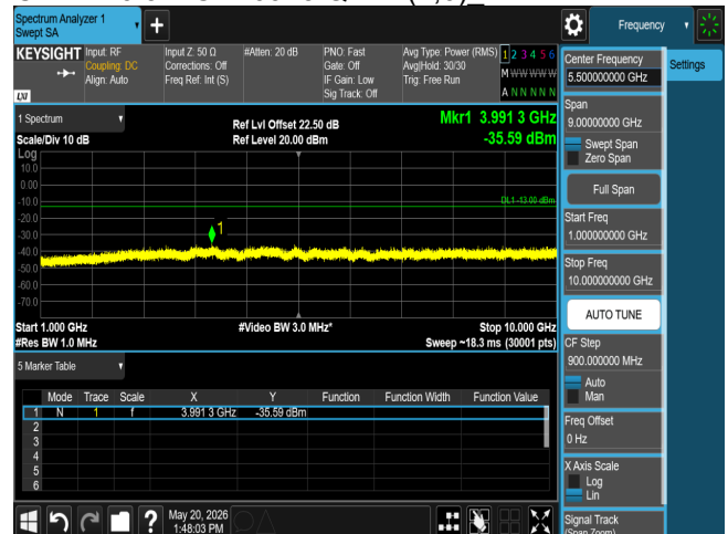
CSE B26 3M CH26915 QPSK(1,0)
