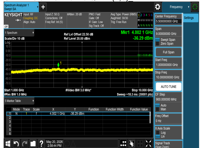
CSE B26 5M CH26740 QPSK(1,0)
