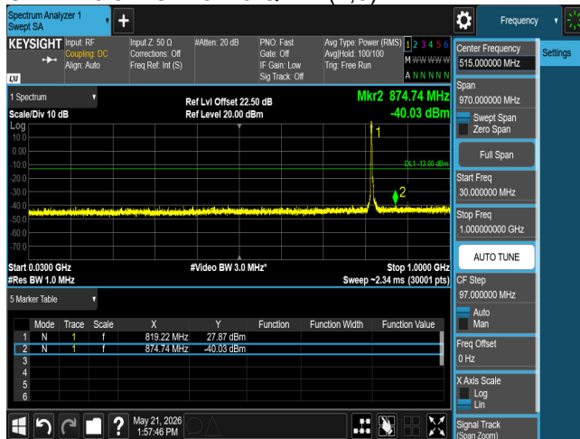
CSE B26 5M CH26740 QPSK(1,0)
