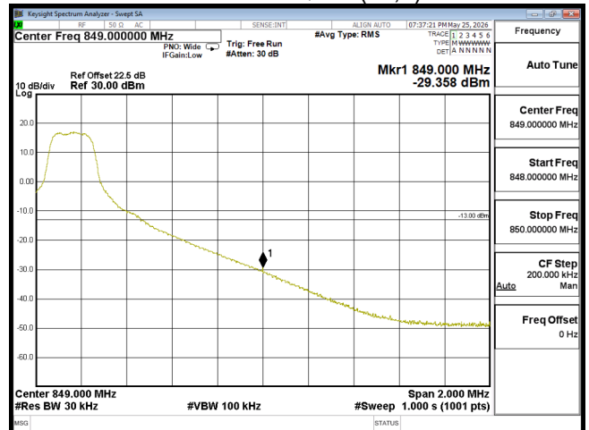
EDGE B26 15M CH26965 QPSK(1,74)
