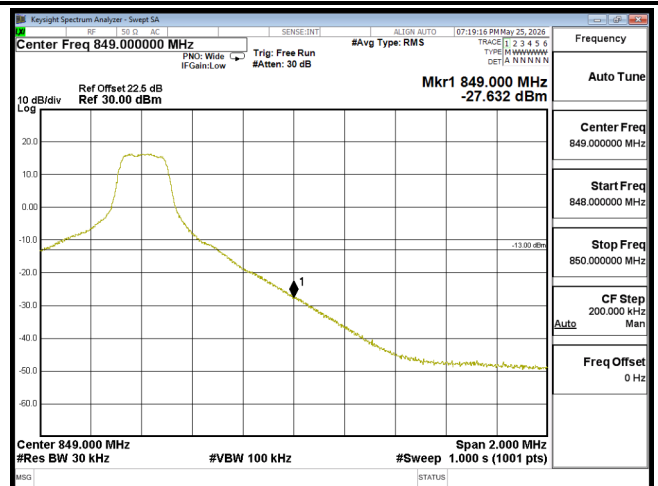
EDGE B26 10M CH26990 QPSK(1,49)
