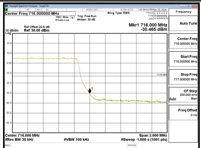
EDGE B12 3M CH23165 QPSK(15,0)
