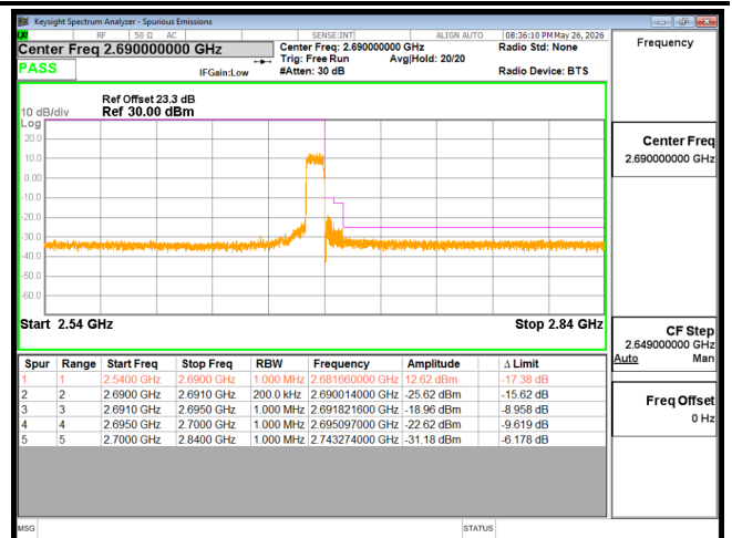
EDGE B41 10M CH41540 QPSK(50,0)
