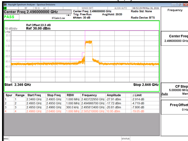
EDGE B41 15M CH39725 QPSK(75,0)
