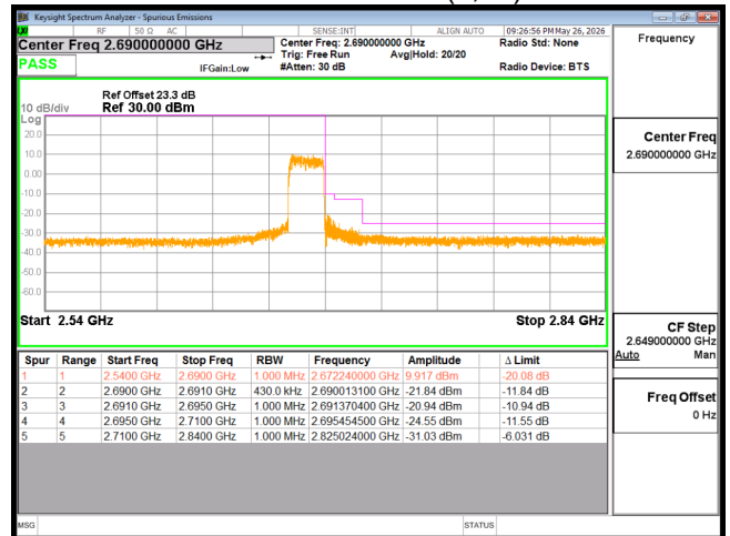
EDGE B41 20M CH41490 QPSK(100,0)
