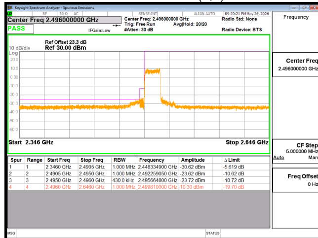
EDGE B41 20M CH39750 QPSK(100,0)
