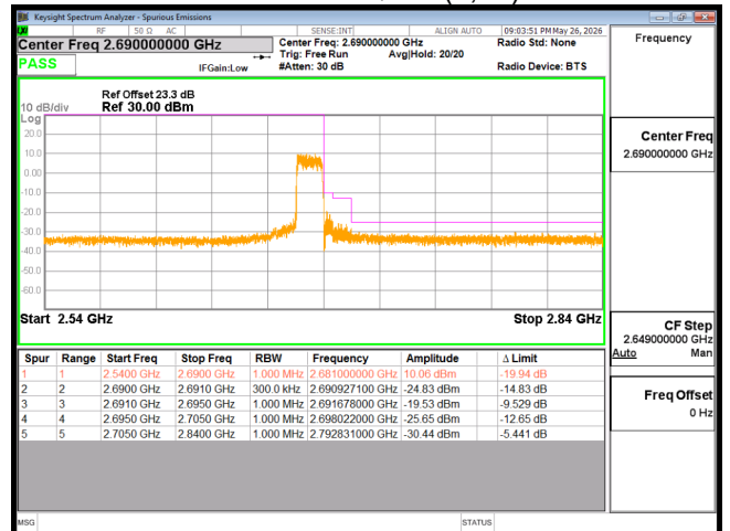
EDGE B41 15M CH41515 QPSK(75,0)
