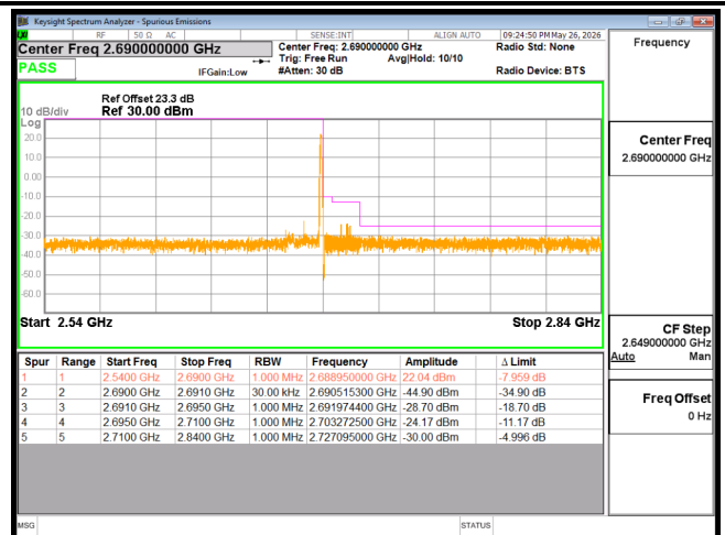
EDGE B41 20M CH41490 QPSK(1,99)
